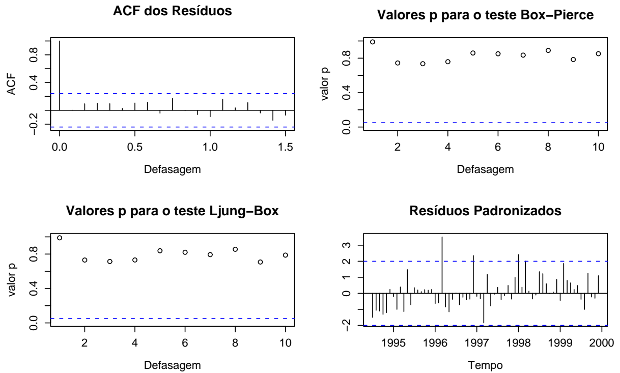
Figura 4.1. Gráficos de diagnóstico do modelo SARIMA(0,0,1) × (1,0,0) para a série IR.dez.99.
