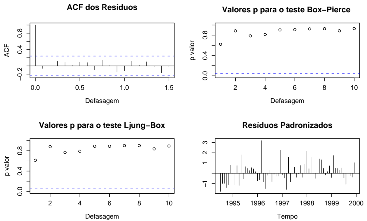
Figura 4.2. Gráficos de diagnóstico do modelo SARIMA(1,0,0) × (1,0,0) para a série log.IR.dez.99.
