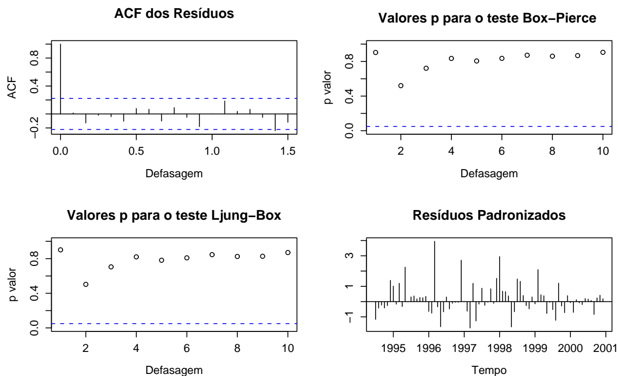
Figura 4.3. Gráficos de diagnóstico do modelo SARIMA(1, 0, 1) × (1, 0, 1) para a série IR.dez.00.
