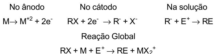
Figura 33. Esquema geral de funcionamento de ânodos de sacrifício.
