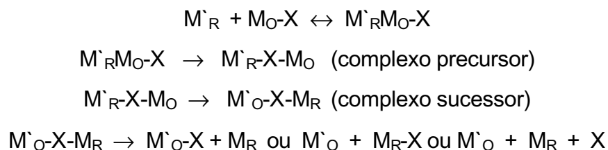
Figura 27: Representação da TE de esfera interna, Mo= Complexo metálico oxidado, M R = Complexo metálico reduzido.
