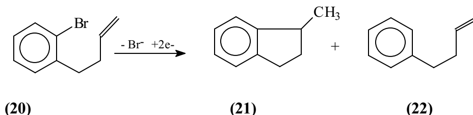
Figura 15. Ciclização catódica do o -3-(butenil)bromobenzeno.
