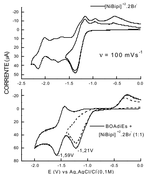
Figura 58: Voltamograma cíclico do [\text{NiBipi}]^{+2} \cdot 2\text{Br}^- em DMF/TBABr (0,1 mol L -1 ), com e sem adição de BOAdiEs em eletrodo de disco de ouro, \nu = 0,1 \text{ V s}^{-1} .
