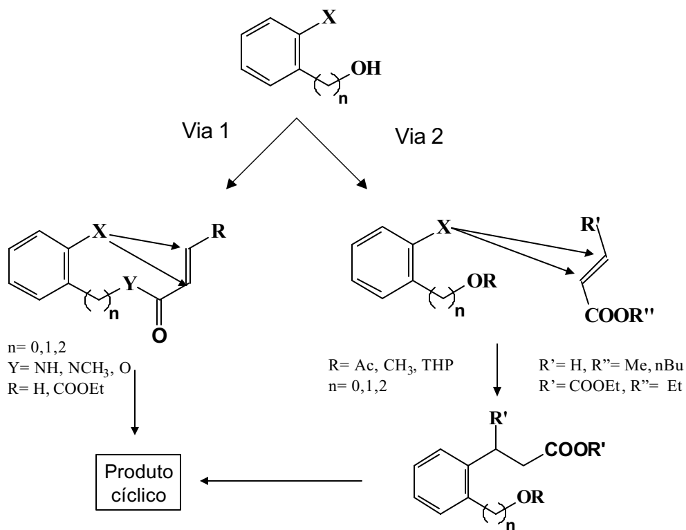
Figura 44. Possibilidades reacionais segundo a via 1 e 2 de síntese.
