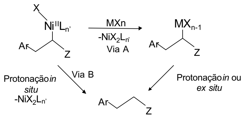
Figura 41. Evidência de transmetalção.
