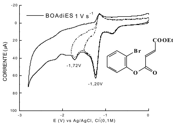
Figura 53. Voltametria cíclica de BOAdiEs em carbono vítreo, DMF/TBABr (0,1 mol L -1 ), \nu = 1 \text{ V s}^{-1} .
