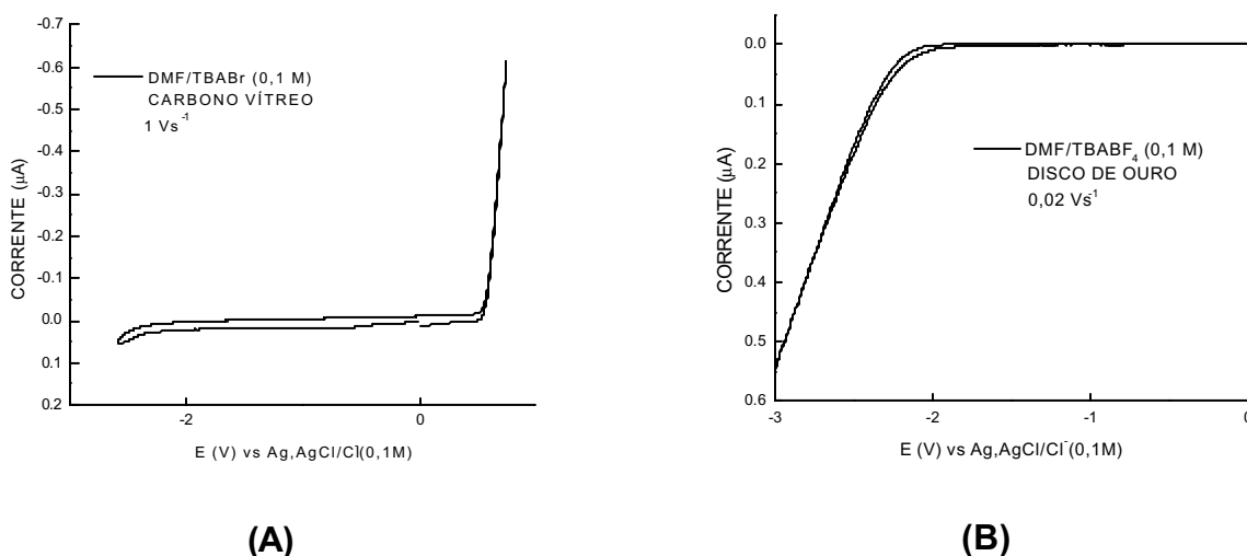
Figura 46: Voltamogramas cíclicos dos ES: (A) DMF/TBABr/Carbono Vítreo; (B) DMF/TBABF 4 /Disco de Ouro.
