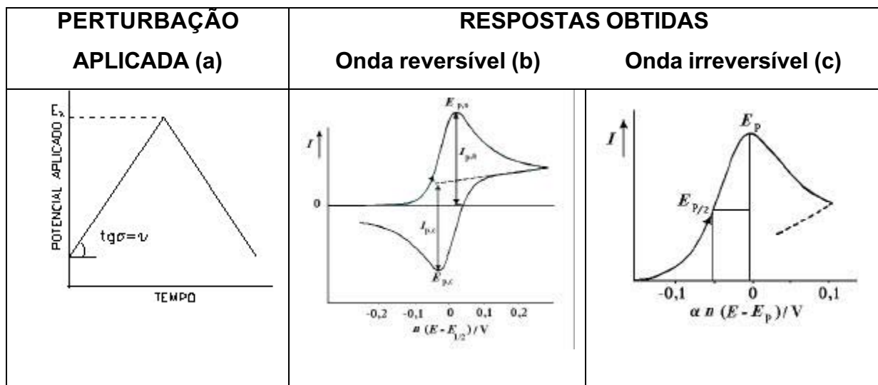
Figura 19. Perturbação aplicada e resultados obtidos em experimentos ciclo voltamétricos.
