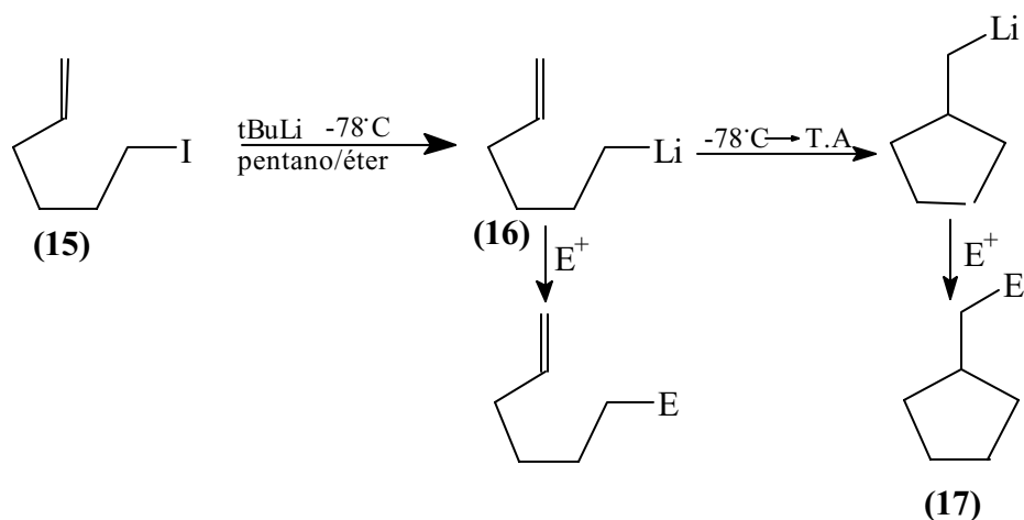
Figura 6. Ciclização intramolecular do 6-iodo-1-hexeno.
