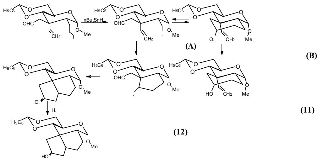
Figura 3. Ataque de radical alquila a grupos aldeídico e olefínico.
