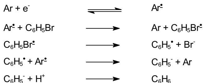
Figura 24. Redução indireta do bromobenzeno, utilizando compostos aromáticos como mediadores.
