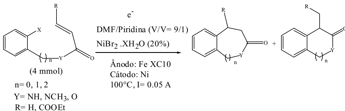
Figura 60. Condições reacionais para tentativas de eletrociclização utilizadas com os precursores
