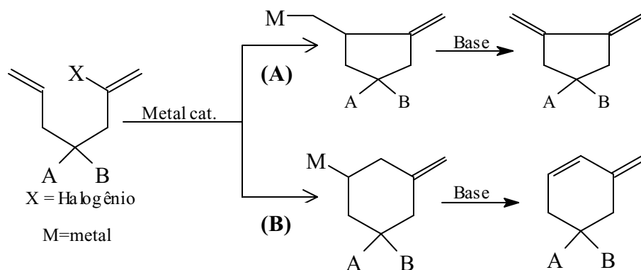
Figura 7. Exemplo de reação de Heck catalisada por paládio.
