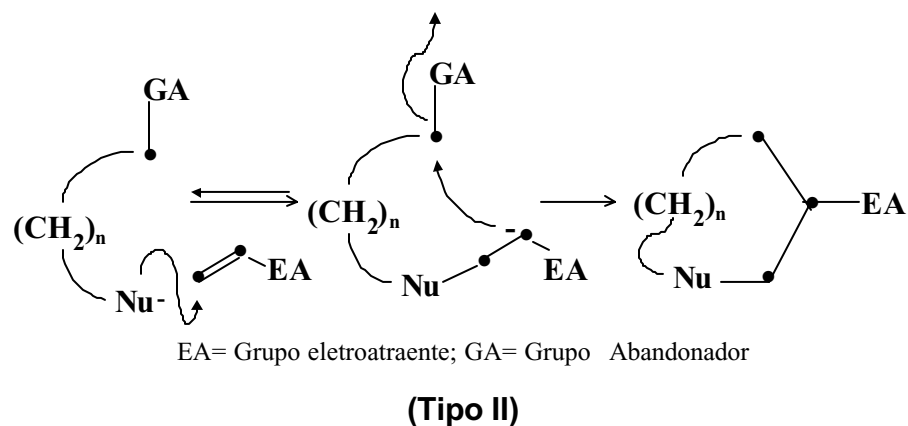
Figura 5. Representação de reações de ciclização iniciadas por adição de Michael (Tipo I e II).
