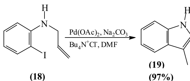
Figura 8. Síntese do metilindol através de reação de Heck.
