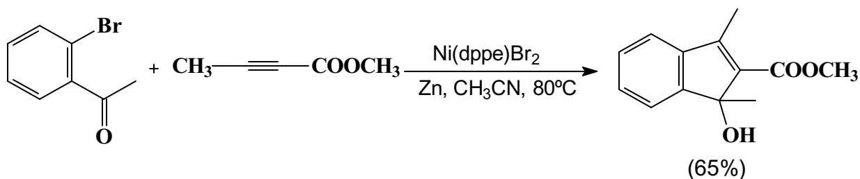
Figura 10. Reação de carbociclização catalisada por complexo de níquel.
