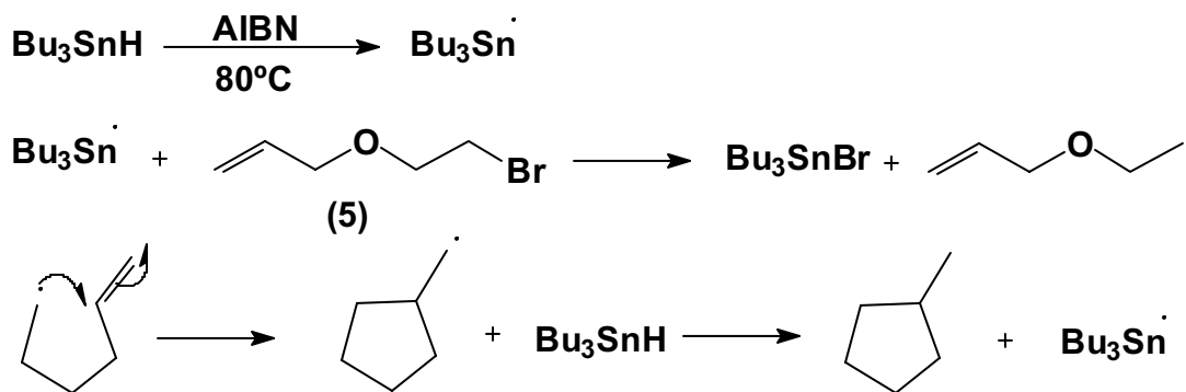
Figura 1. Ciclização radicalar do 3 (2-bromo-1-etoxi) propeno (5) utilizando AIBN e hidreto de tributilestanho.
