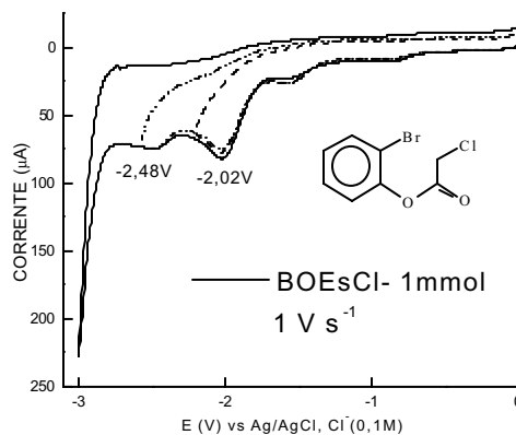
Figura 55. Voltametria cíclica de BOEsCl em carbono vítreo, DMF/TBABr (0,1 mol L -1 ) \nu = 1 \text{ V s}^{-1} .
