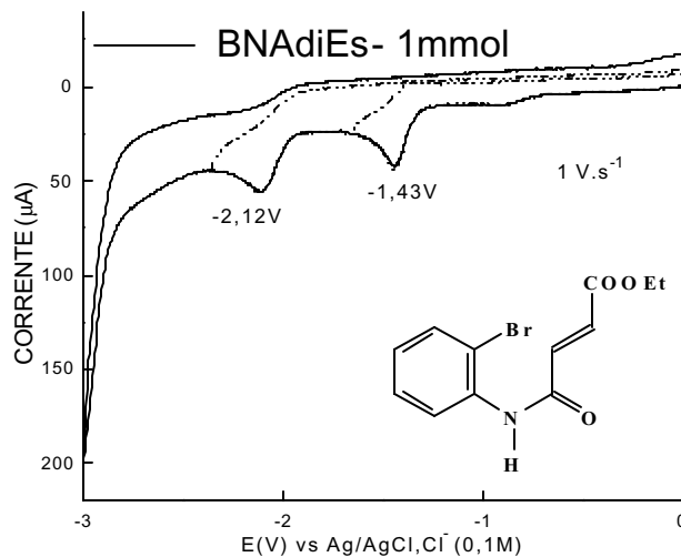
Figura 54. Voltametria cíclica de BNAdiEs em carbono vítreo, DMF/TBABr (0,1 mol L -1 ), \nu = 1 \text{ V s}^{-1} .
