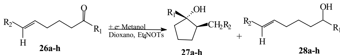
Figura 17. Redução direta do grupo carbonila de cetonas olefinicas não conjugadas.
