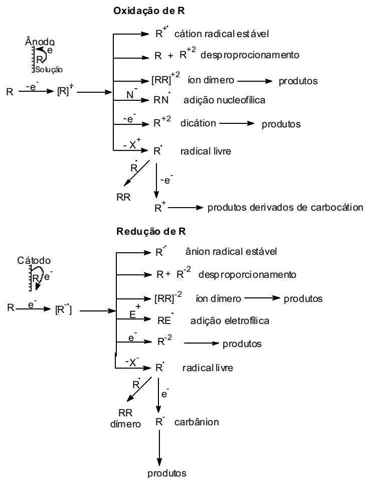
Figura 12. Intermediários reativos formados durante o processo eletroquímico.
