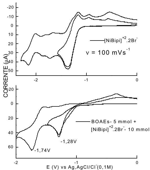
Figura 57: Voltamograma cíclico do [\text{NiBipi}]^{+2} \cdot 2\text{Br}^- em DMF/TBAPF 4 (0,1 mol L -1 ), com e sem adição de BOAdiEs. em eletrodo de disco de ouro - 1,5 mm 2 , \nu = 0,1 \text{ V/s} .
