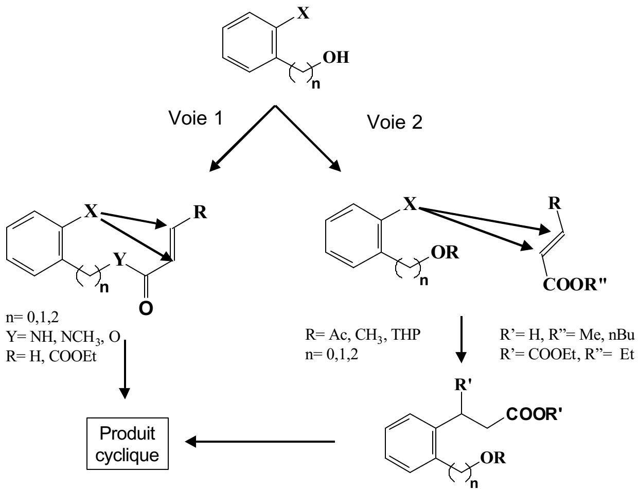
Figure 2. Schéma des deux voies de synthèse étudiées.
