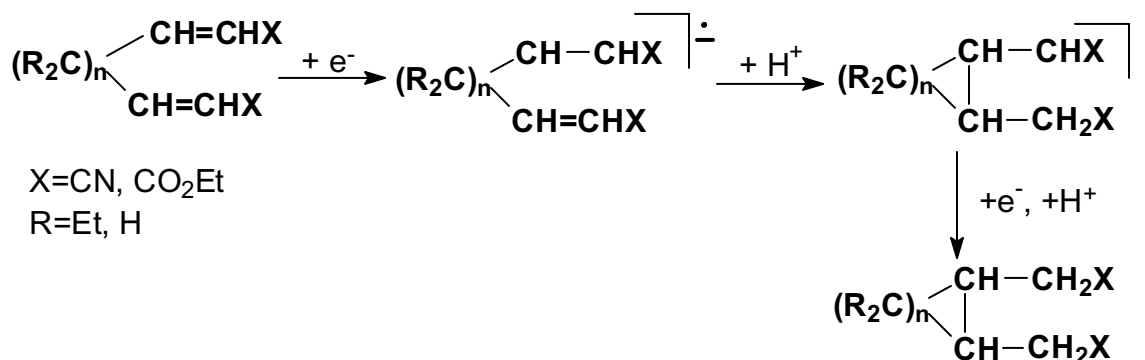
Figura 13. Reação de eletroidroclicização.
