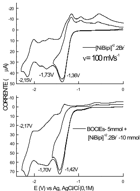
Figura 59: Voltamograma cíclico do [\text{NiBipi}]^{2+} \cdot 2\text{Br}^- em DMF/TBABr (0,1 mol L -1 ), com e sem adição de BOCIEs em eletrodo de disco de ouro, v = 0,1 \text{ V s}^{-1} .
