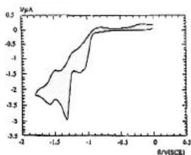
Figura 32. Voltamograma cíclico [\text{NiBipi}]^{+2}\cdot 2\text{Br}^- em \text{DMF}/\text{TBABF}_4 em eletrodo de ouro com adição sucessiva de 2-bromo-2-buteno.
