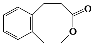
Figura 65. Lactona de 8 membros (XXXII) obtida do intermediário XXI, pela via 2 de síntese.
