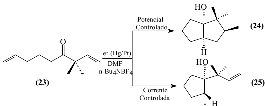
Figura 16. Redução catódica da dienona não conjugada.
