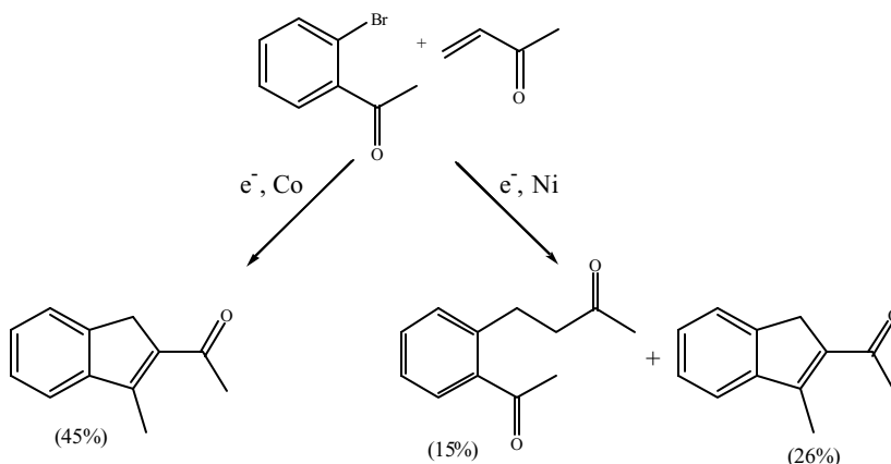
Figura 39. Formação de produto cíclico durante eletroacoplamento catalisado por níquel e cobalto.
