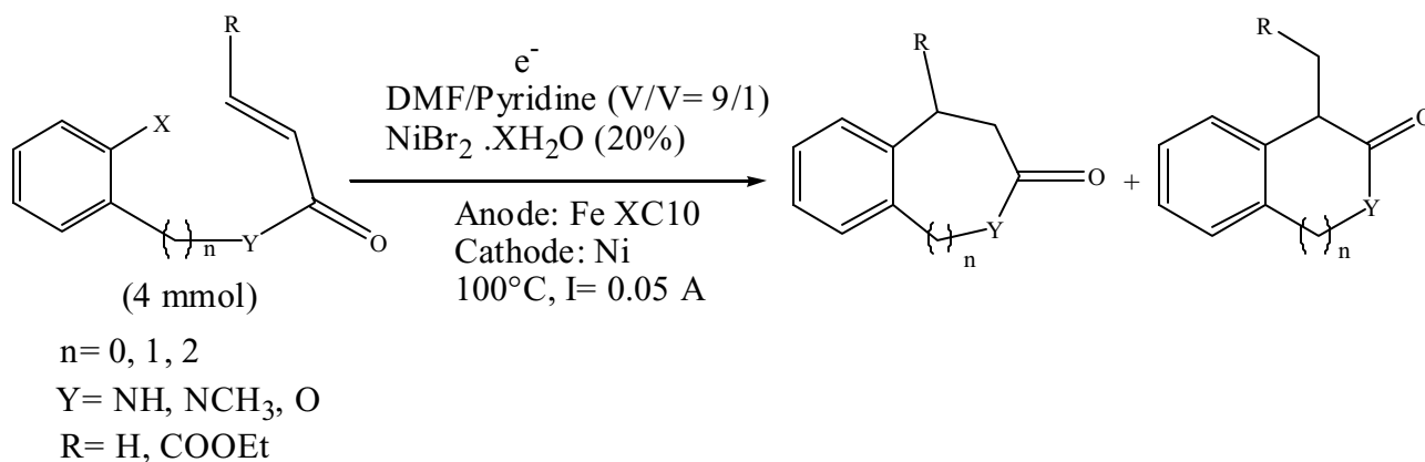
Figure 4. Les meilleur conditions réactionnelles adoptés.
