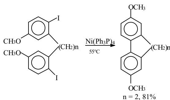
Figura 9. Síntese de orto -bifenilas catalisada por complexo de níquel.
