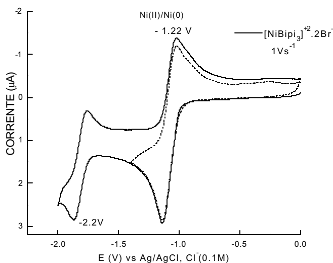
Figura 49. Voltamograma cíclico do [NiBipi 3 ] +2 .2Br - (excesso de bipyridina) em DMF/TBABF 4 (0,1 mol L -1 ) em eletrodo de ouro - 0,25 mm 2 , \nu = 1 V/s.
