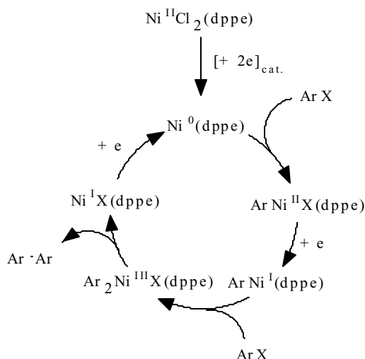
Figura 34. Acoplamento de haletos aromáticos catalisado por complexo de Níquel.
