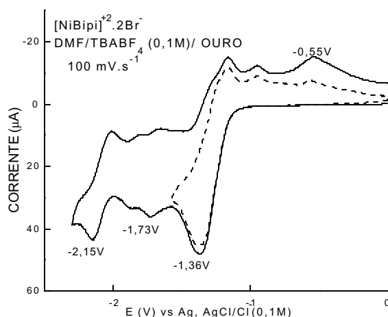
Figura 48. Voltamograma cíclico do complexo [\text{NiBipi}]^{+2} \cdot 2\text{Br}^- em \text{DMF/TBABF}_4 (0,1 mol.L -1 ) em eletrodo de ouro - 1,5 mm 2 , v = 100 mV/s.
