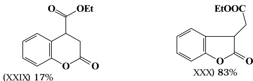
Figura 63. Produtos cíclicos obtidos do precursor XV.
