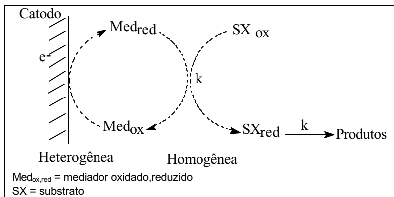
Figura 20. Princípio da eletrólise indireta (redução).
