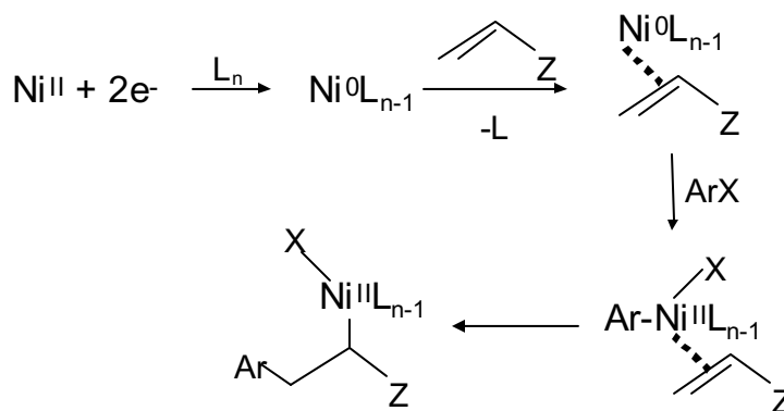
Figura 40. Mecanismo de arilação eletroquímica de olefina ativada
