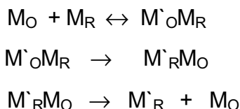
Figura 26: Representação da TE de esfera externa, Mo= Complexo metálico oxidado, M R = Complexo metálico reduzido.
