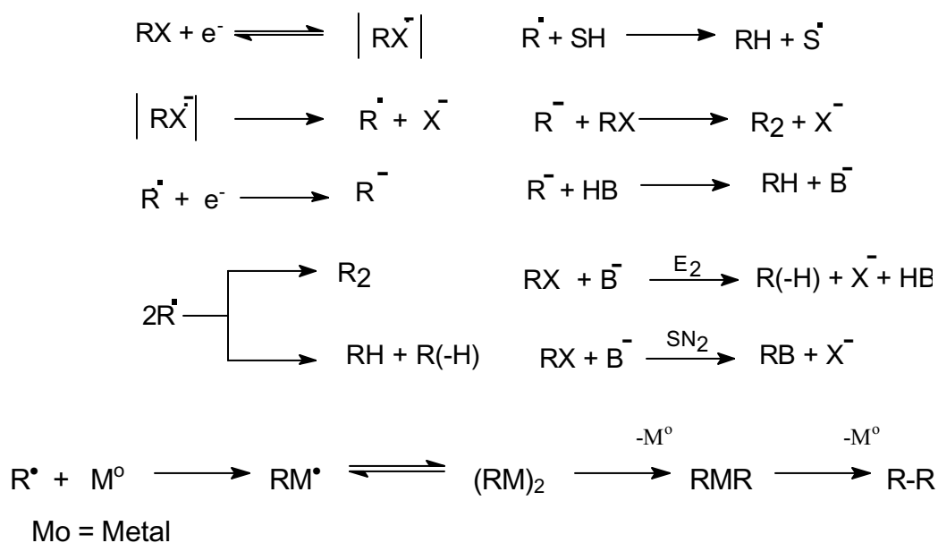
Figura 22. Possibilidades mecanísticas na redução de monoalotos de alquila.
