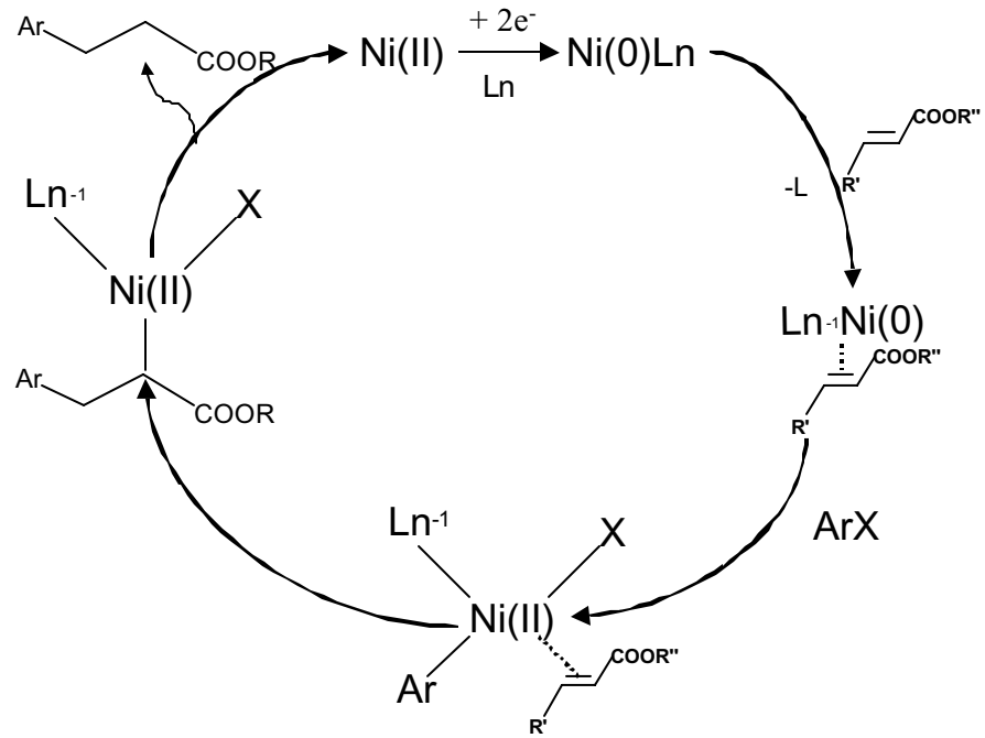
Figura 67. Provável ciclo catalítico no processo de eletroacoplamento de olefinas a haletos aromáticos.
