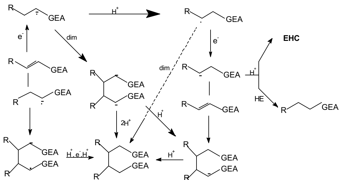
Figura 25. Esquema reacional típico para a redução de olefinas ativadas.
