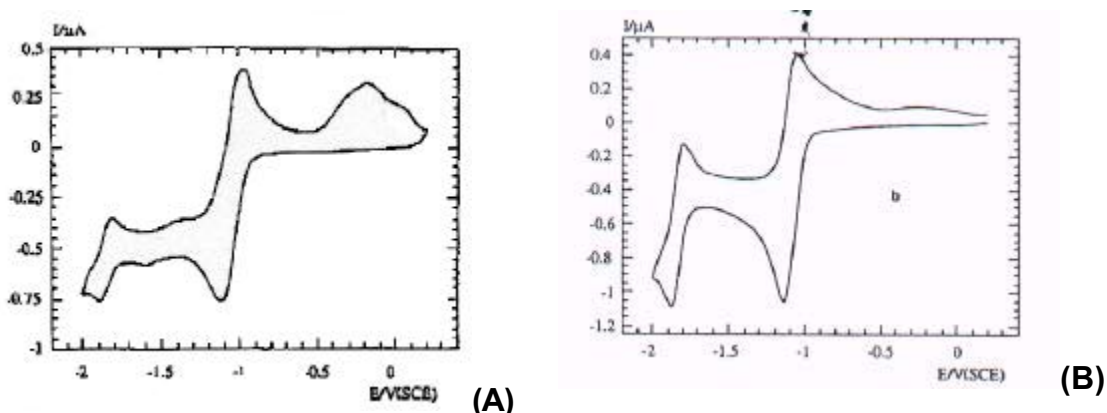
Figura 31. Voltamograma cíclico [\text{NiBipi}]^{+2}\cdot 2\text{Br}^- em \text{DMF}/\text{TBABF}_4 (A), em eletrodo de ouro, (B): [\text{NiBipi}_3]^{+2}\cdot 2(\text{BF}_4)^- em \text{DMF}/\text{TBABF}_4 e microeletrodo de ouro, 0,25\text{mm}^2 .
