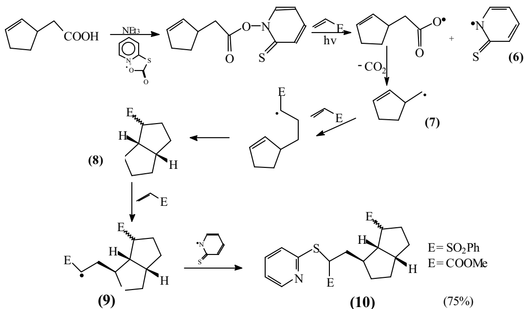
Figura 2. Exemplo de reação cascata (tandem).
