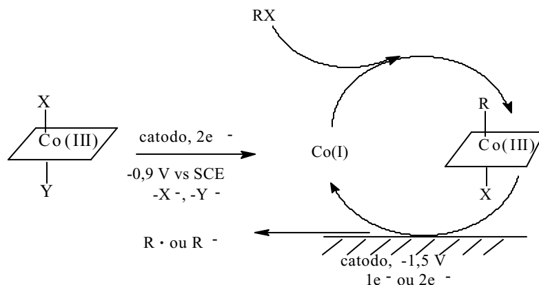
Figura 21. Redução catalítica de haletos orgânicos em presença da vitamina B 12 .
