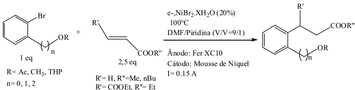
Figura 62. Condições reacionais aplicadas nas reações de eletroacoplamento bimolecular da via 2 de síntese
