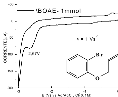
Figura 51. Voltametria cíclica de BOAE em carbono vítreo, DMF/TBABr (0,1 mol L -1 ), v = 1 \text{ V s}^{-1} .
