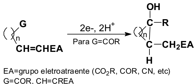
Figura 14. Processo geral CER.
