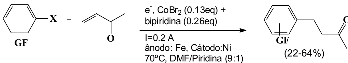
Figura 38. Eletroacoplamento catalisado por complexos de cobalto
