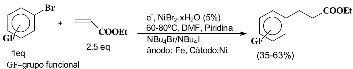
Figura 37. Eletroacoplamento catalisado por complexos de níquel.
