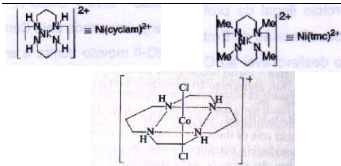
Figura 28. Fórmulas de alguns complexos de níquel e cobalto escolhidos.
