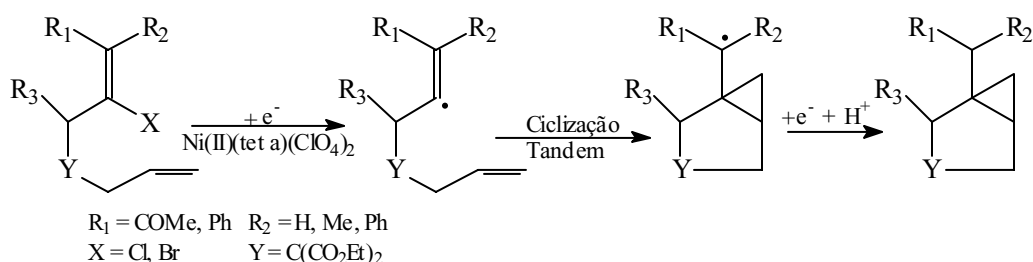
Figura 36. Preparação de ciclopropanos bicíclicos e tricíclicos.
