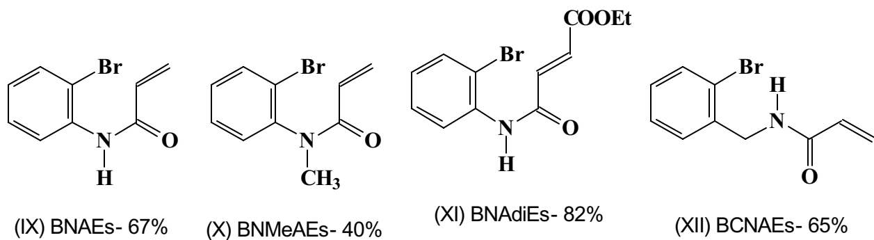
Figure 3. Précurseurs synthésés et utilisés pour la voie 1, avec les rendements respectifs (A) série oxygénée et (B) série azotée.
