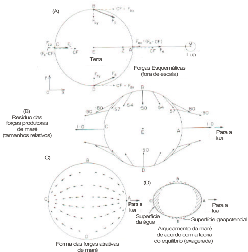
Figura 04. (A) direção esquemática das forças centrípetas (CF) e gravitacional da lua por unidade de massa ( F_a , F_b , F_c , F_d ) em pontos na Terra, (B) direção e magnitudes relativas dos resíduos de CF e F em pontos da superfície terrestre, (C) forma das forças atrativas horizontais na superfície da Terra, (D) arqueamento da maré (muito exagerado) em A e C de acordo com a teoria do equilíbrio para o oceano cobrindo toda a Terra (Pond & Pickard, 1983).
