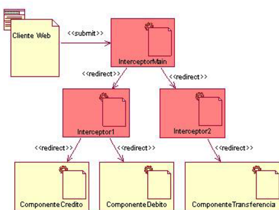
Figura 2.2: Exemplo de uma cadeia de Interceptadores.
