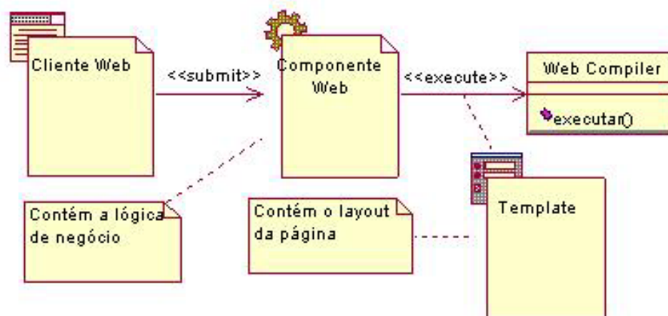
Figura 2.14: Estrutura do padrão Web Compiler .
