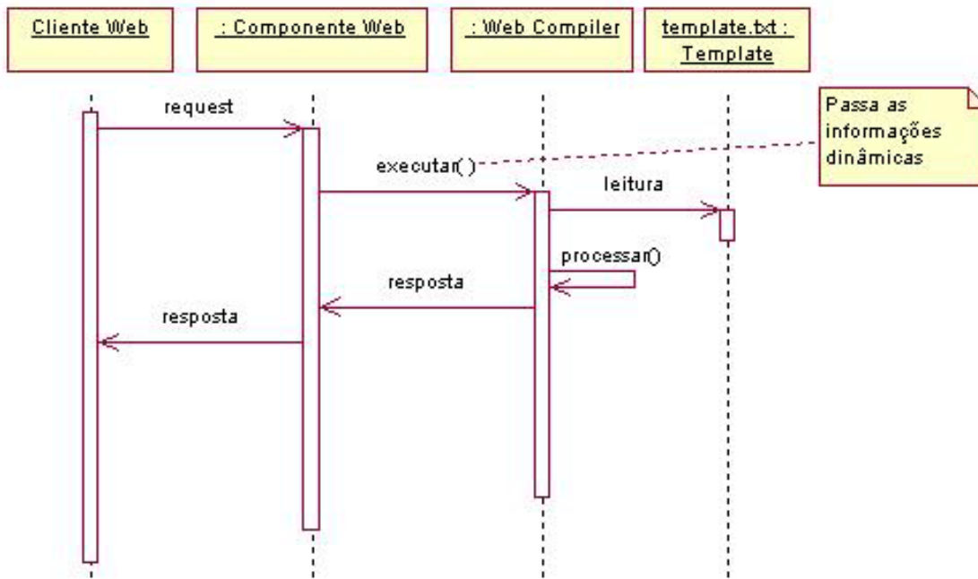
Figura 2.15: Diagrama de seqüência dos componentes do padrão Web Compiler .
