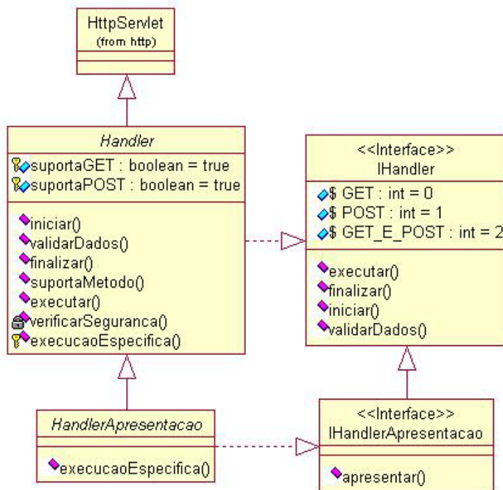
Figura 3.4: Diagrama das classes básicas do framework relacionadas com os handlers de apresentação.
