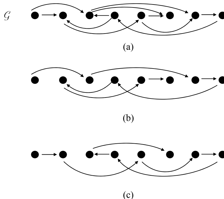
Figura 17: (a) Grafo \mathcal{G} para o espectro \Gamma com dois Caminhos Hamiltonianos correspondendo às seqüências (b) ATGCGTGGCA e (c) ATGGCGTGCA. Adaptado de (PEVZNER, 2000).
