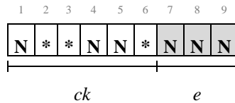
Figura 4. Esquema de um probe para c = 2 , k = 3 e e = 3 .
