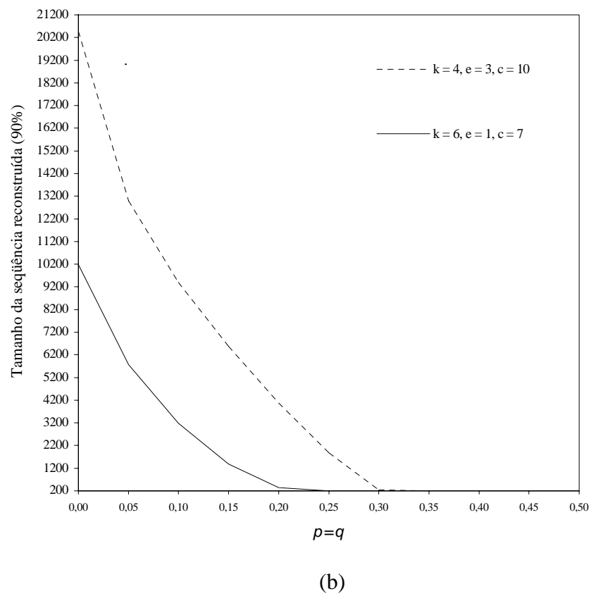
Figura 27A: Tamanho da seqüência corretamente reconstruída em aproximadamente 90% dos casos versus as taxas p e q ( p = q ) de erros, quando k + e = 7 , ck + e = 43 , (a) n = 4^8 e (b) n = 4^9 .
