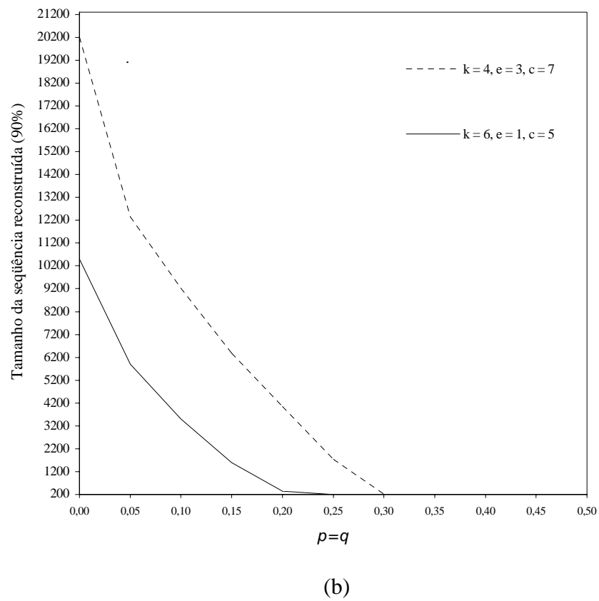
Figura 24A: Tamanho da seqüência corretamente reconstruída em aproximadamente 90% dos casos versus as taxas p e q ( p = q ) de erros, quando k + e = 7 , p = 0 , ck + e = 31 , (a) n = 4^8 e (b) n = 4^9 .
