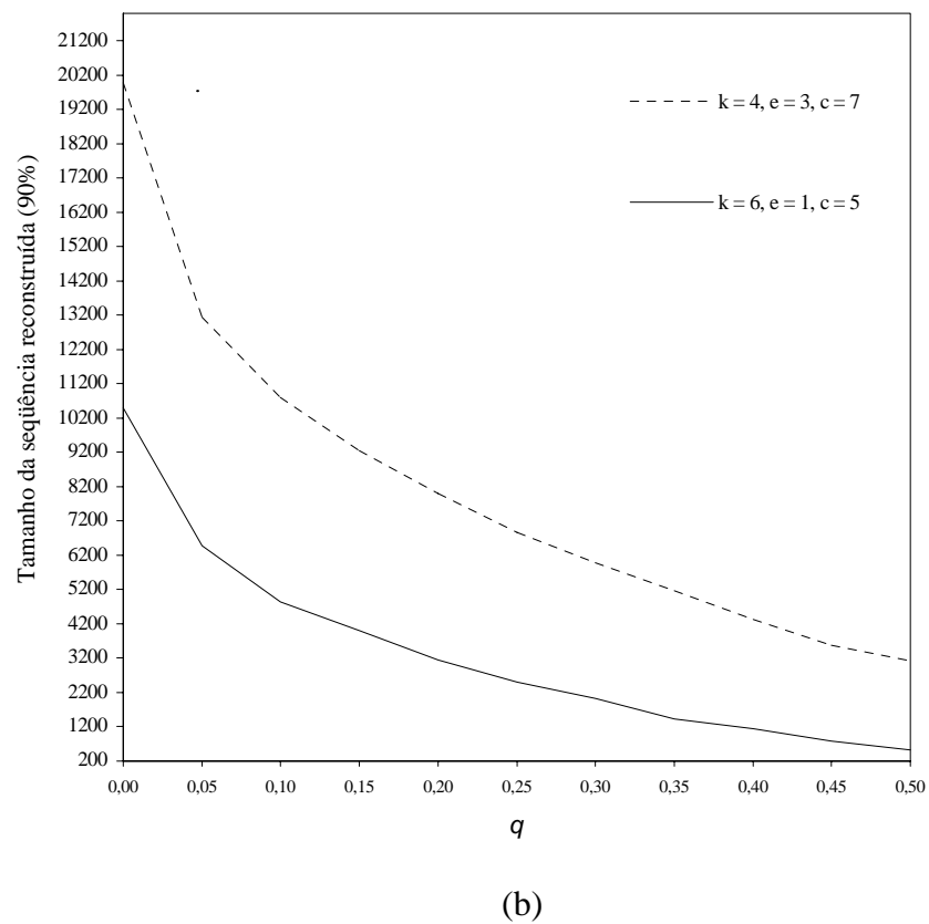
Figura 23A: Tamanho da seqüência corretamente reconstruída em aproximadamente 90% dos casos versus a taxa q de erro falso negativo, quando k + e = 7 , p = 0 , ck + e = 31 , (a) n = 4^8 e (b) n = 4^9 .
