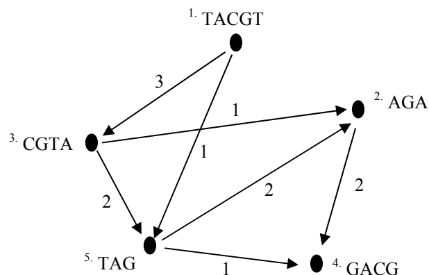
Figura 13: Exemplo de um grafo de sobreposição para os fragmentos da Figura 9.
