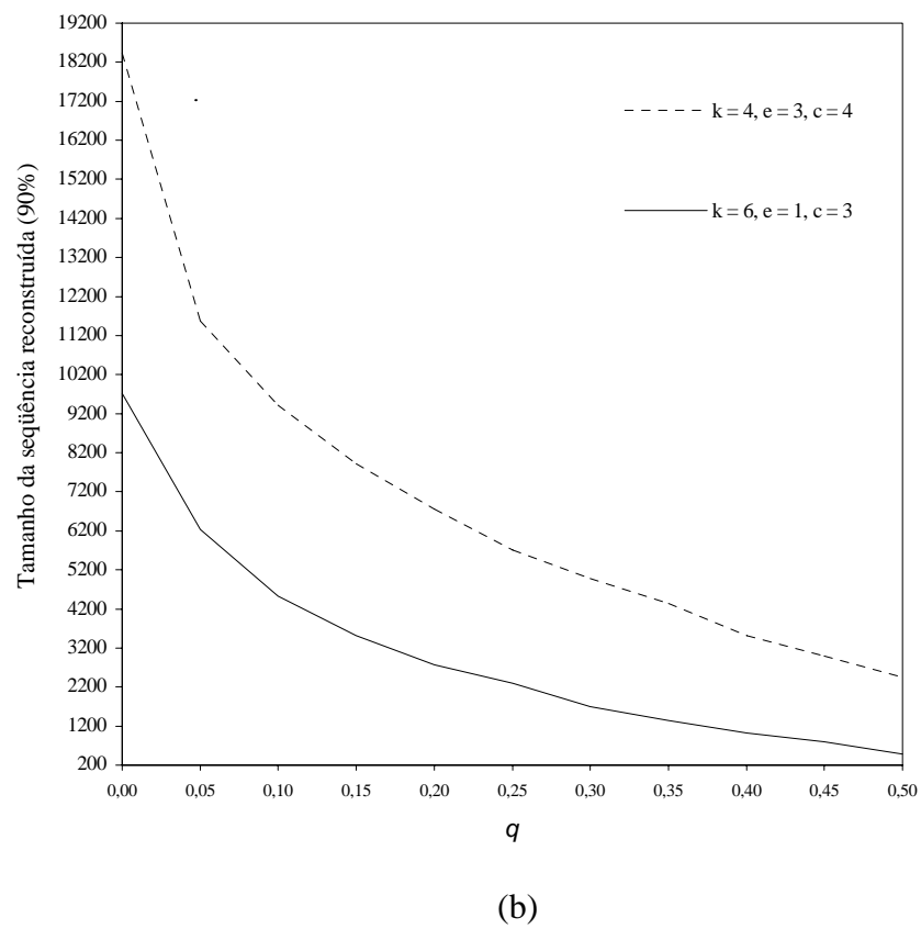
Figura 20A: Tamanho da seqüência corretamente reconstruída em aproximadamente 90% dos casos versus a taxa q de erro falso negativo, quando k + e = 7 , p = 0 , ck + e = 19 , (a) n = 4^8 e (b) n = 4^9 .
