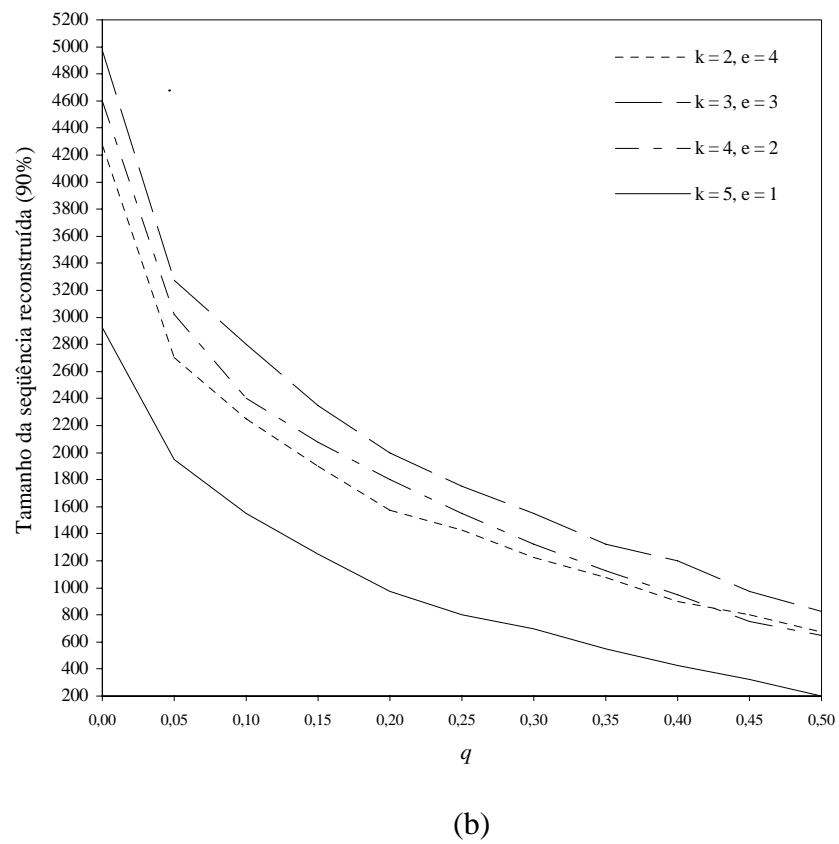
Figura 8A: Tamanho da seqüência corretamente reconstruída em aproximadamente 90% dos casos versus a taxa q de erro falso negativo, quando k + e = 6 , p = 0 , c = 10 , (a) n = 4^7 e (b) n = 4^8 .
