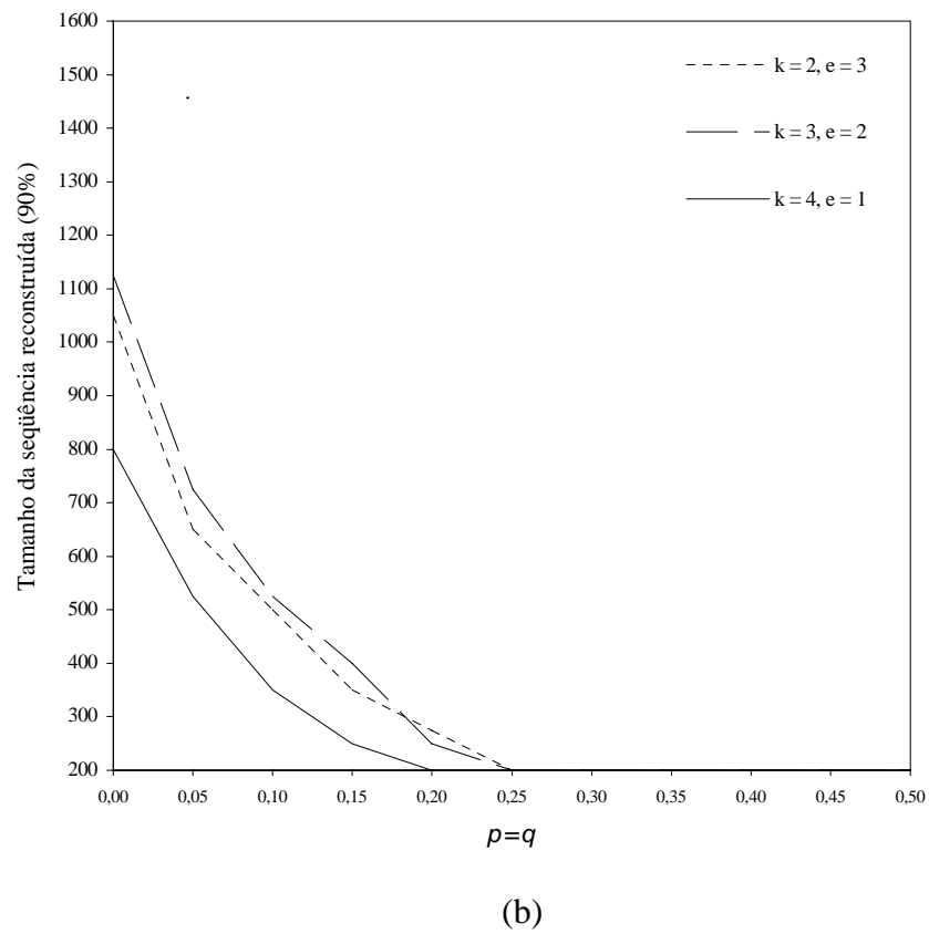
Figura 6A: Tamanho da seqüência corretamente reconstruída em aproximadamente 90% dos casos versus as taxas p e q ( p = q ) de erros, quando k + e = 5 , c = 10 , (a) n = 4^6 e (b) n = 4^7 . Em (a), a linha (k = 4, e = 1) é menor que 200.
