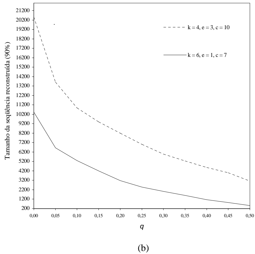
Figura 26A: Tamanho da seqüência corretamente reconstruída em aproximadamente 90% dos casos versus a taxa q de erro falso negativo, quando k + e = 7 , p = 0 , ck + e = 43 , (a) n = 4^8 e (b) n = 4^9 .
