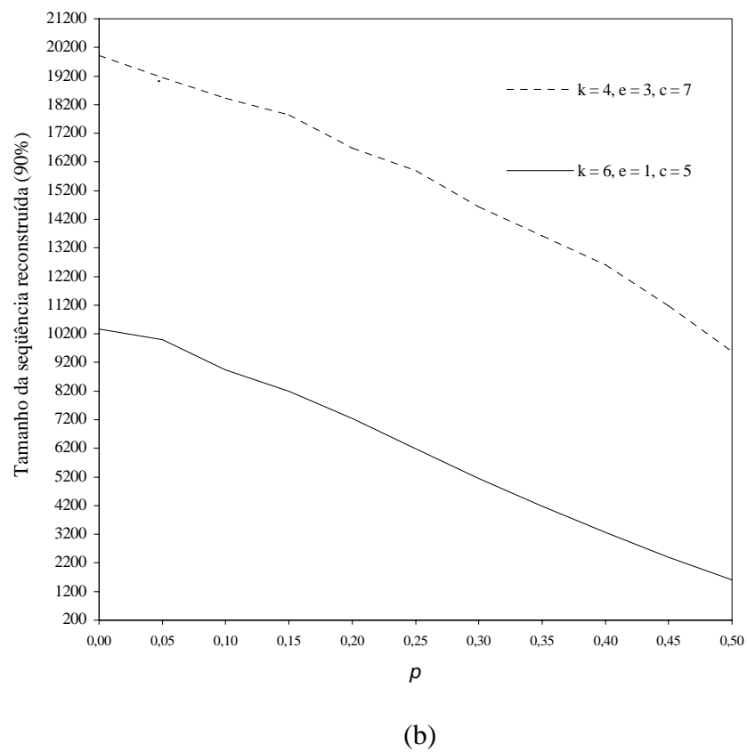
Figura 22A: Tamanho da seqüência corretamente reconstruída em aproximadamente 90% dos casos versus a taxa p de erro falso positivo, quando k + e = 7 , q = 0 , ck + e = 31 , (a) n = 4^8 e (b) n = 4^9 .
