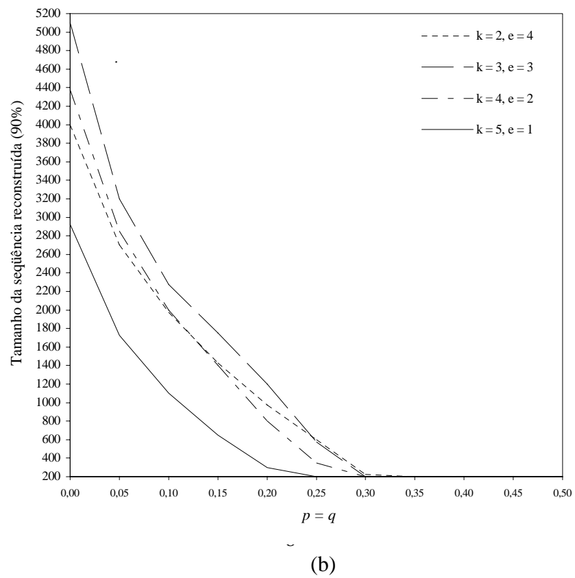
Figura 9A: Tamanho da seqüência corretamente reconstruída em aproximadamente 90% dos casos versus as taxas p e q ( p = q ) de erros, quando k + e = 6 , c = 10 , (a) n = 4^7 e (b) n = 4^8 .
