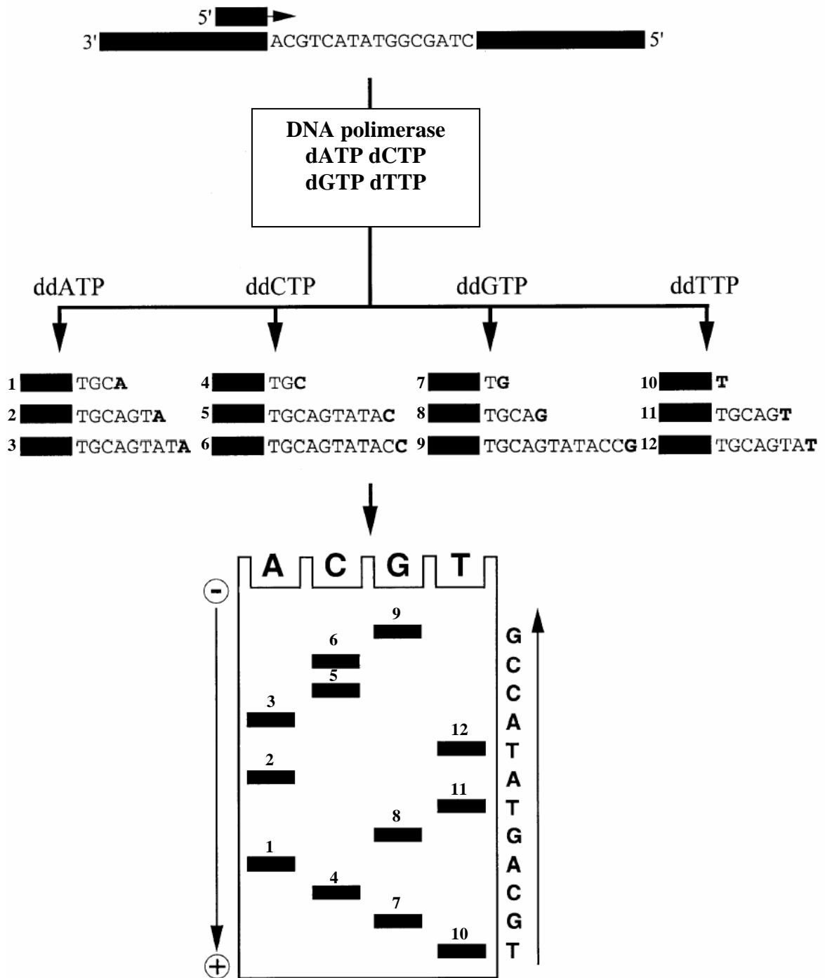
Figura 7: Esquema de funcionamento do método de Terminação de Cadeia de Sanger. Adaptado de (STERKY; LUNDEBERG, 2000).
