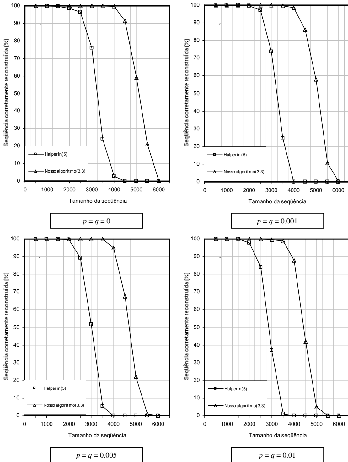
Figura 8. Desempenho do nosso algoritmo e do algoritmo B.
