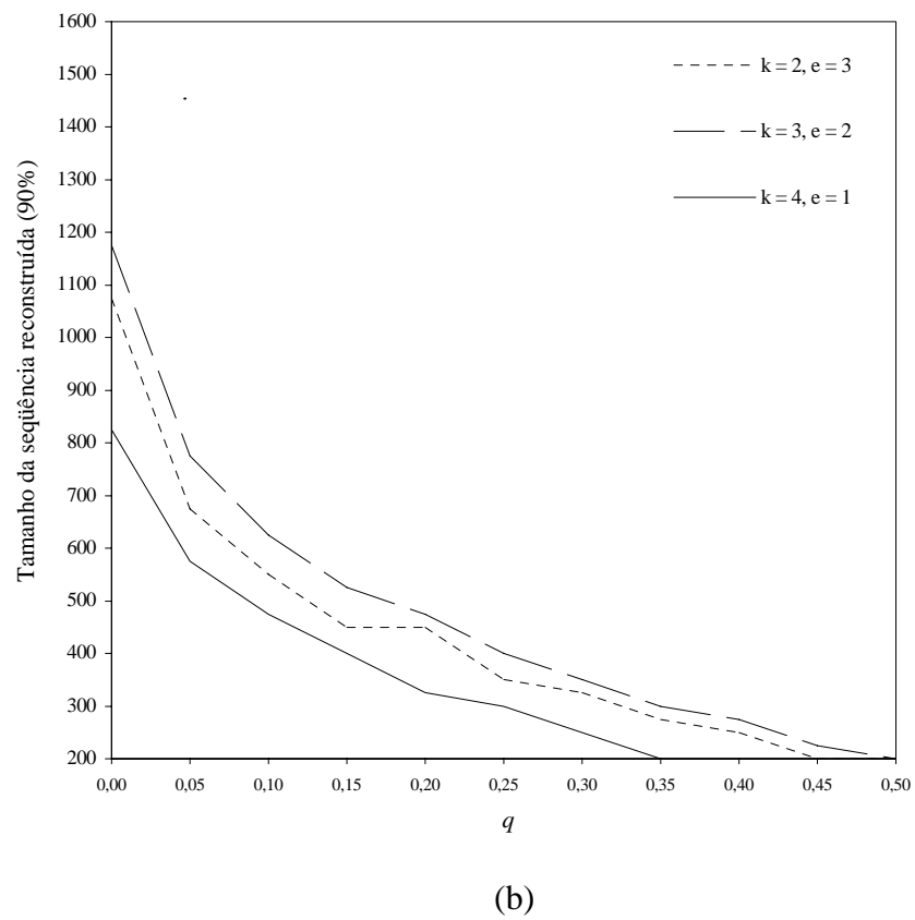
Figura 5A: Tamanho da seqüência corretamente reconstruída em aproximadamente 90% dos casos versus a taxa q de erro falso negativo, quando k + e = 5 , p = 0 , c = 10 , (a) n = 4^6 e (b) n = 4^7 . Em (a), a linha ( k = 4, e = 1 ) é menor que 200.
