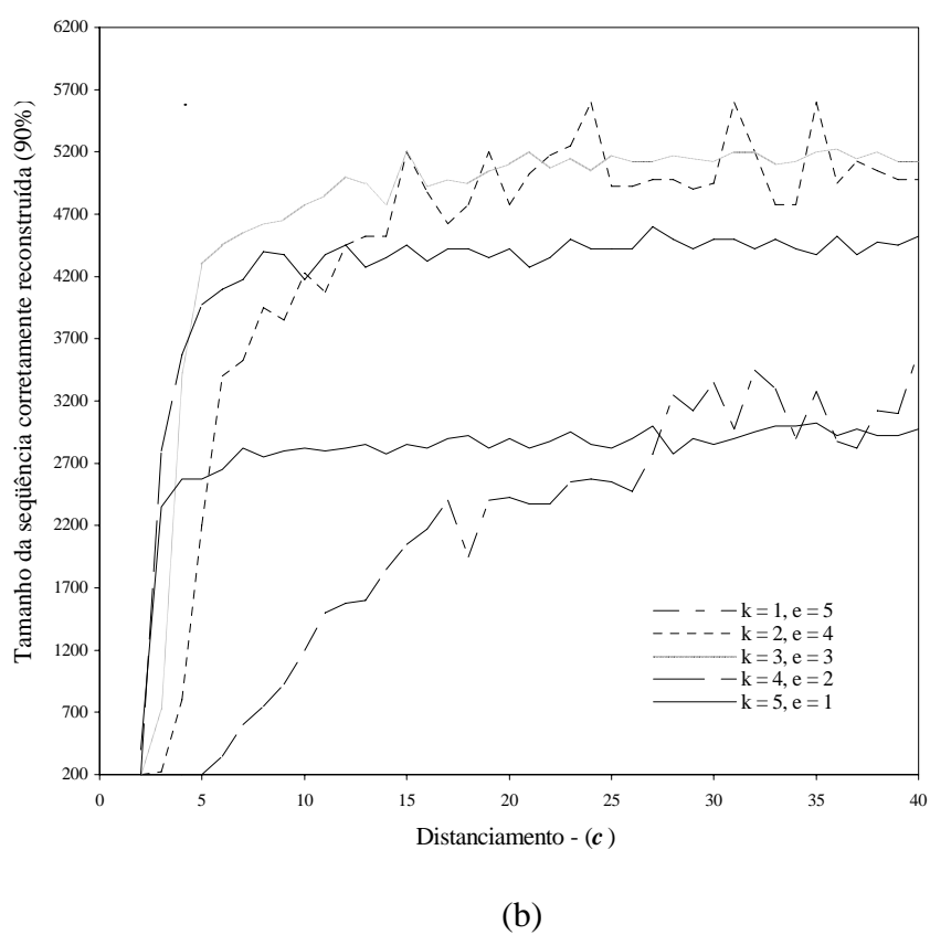
Figura 2A: Tamanho da seqüência corretamente reconstruída em aproximadamente 90% dos casos versus o distanciamento c das bases naturais, quando k + e = 6 , p = q = 0 , (a) n = 4^7 e (b) n = 4^8 .
