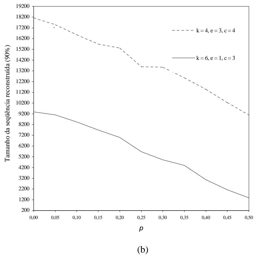
Figura 19A: Tamanho da seqüência corretamente reconstruída em aproximadamente 90% dos casos versus a taxa p de erro falso positivo, quando k + e = 7 , q = 0 , ck + e = 19 , (a) n = 4^8 e (b) n = 4^9 .
