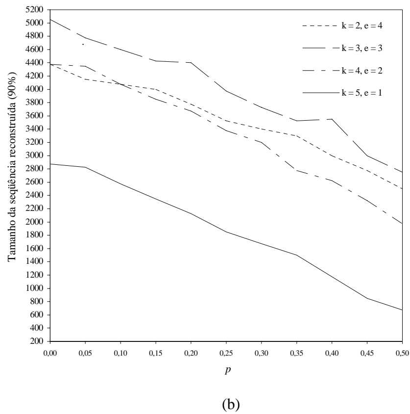
Figura 7A: Tamanho da seqüência corretamente reconstruída em aproximadamente 90% dos casos versus a taxa p de erro falso positivo, quando k + e = 6 , q = 0 , c = 10 , (a) n = 4^7 e (b) n = 4^8 .
