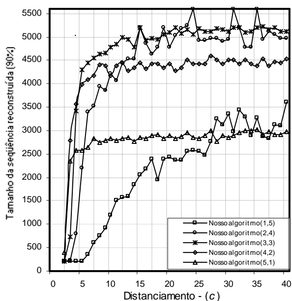
Figura 7. Desempenho do nosso algoritmo para k + e = 6 .
