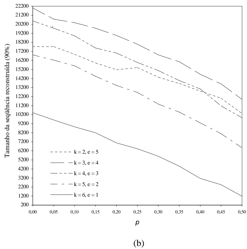
Figura 10A: Tamanho da seqüência corretamente reconstruída em aproximadamente 90% dos casos versus a taxa p de erro falso positivo, quando k + e = 7 , q = 0 , c = 10 , (a) n = 4^8 e (b) n = 4^9 .
