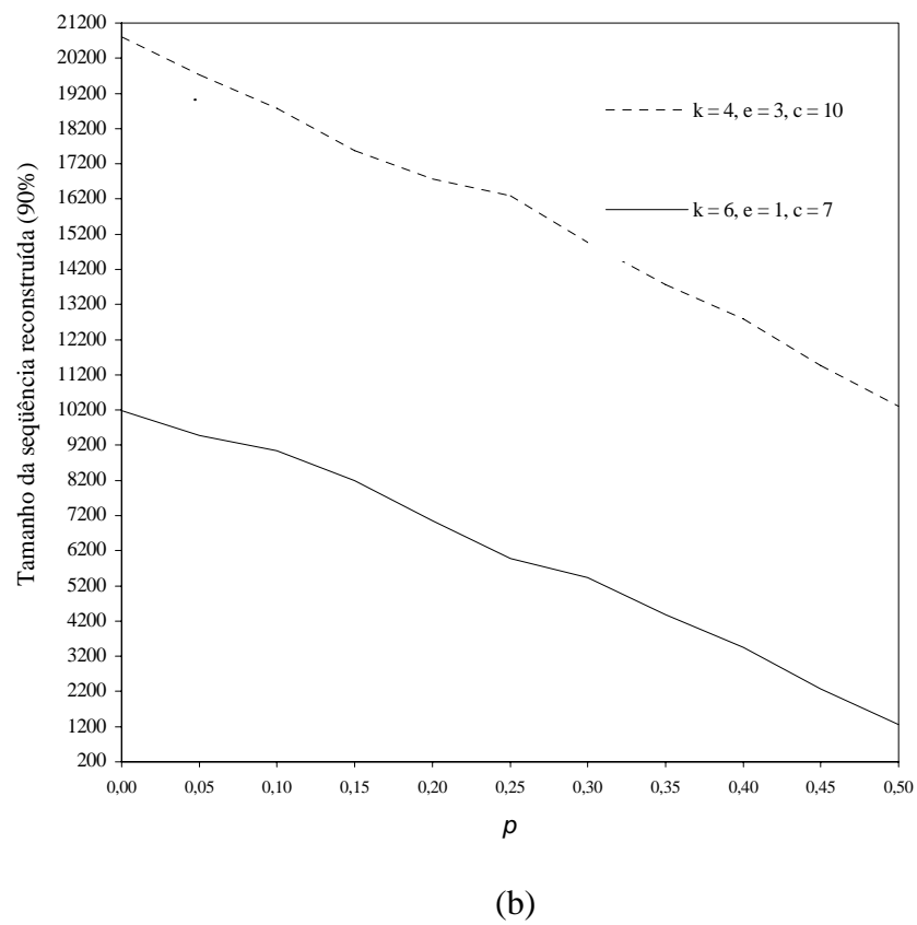
Figura 25A: Tamanho da seqüência corretamente reconstruída em aproximadamente 90% dos casos versus a taxa p de erro falso positivo, quando k + e = 7 , q = 0 , ck + e = 43 , (a) n = 4^8 e (b) n = 4^9 .
