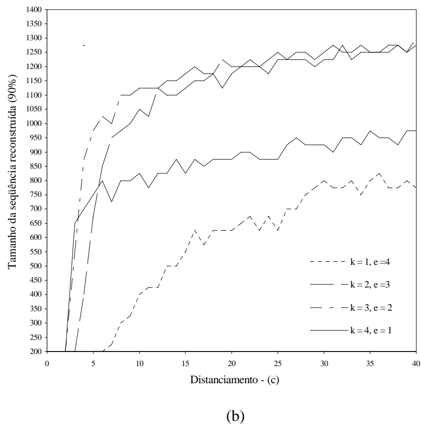
Figura 1A: Tamanho da seqüência corretamente reconstruída em aproximadamente 90% dos casos versus o distanciamento c das bases naturais, quando k + e = 5 , p = q = 0 , (a) n = 4^6 e (b) n = 4^7 .
