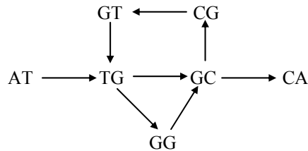
Figura 18: Construção do grafo proposto por Pevzner para o espectro \Gamma = \{ATG, TGG, TGC, GTG, GGC, GCA, GCG, CGT\} . Extraído de (PEVZNER, 2000).
