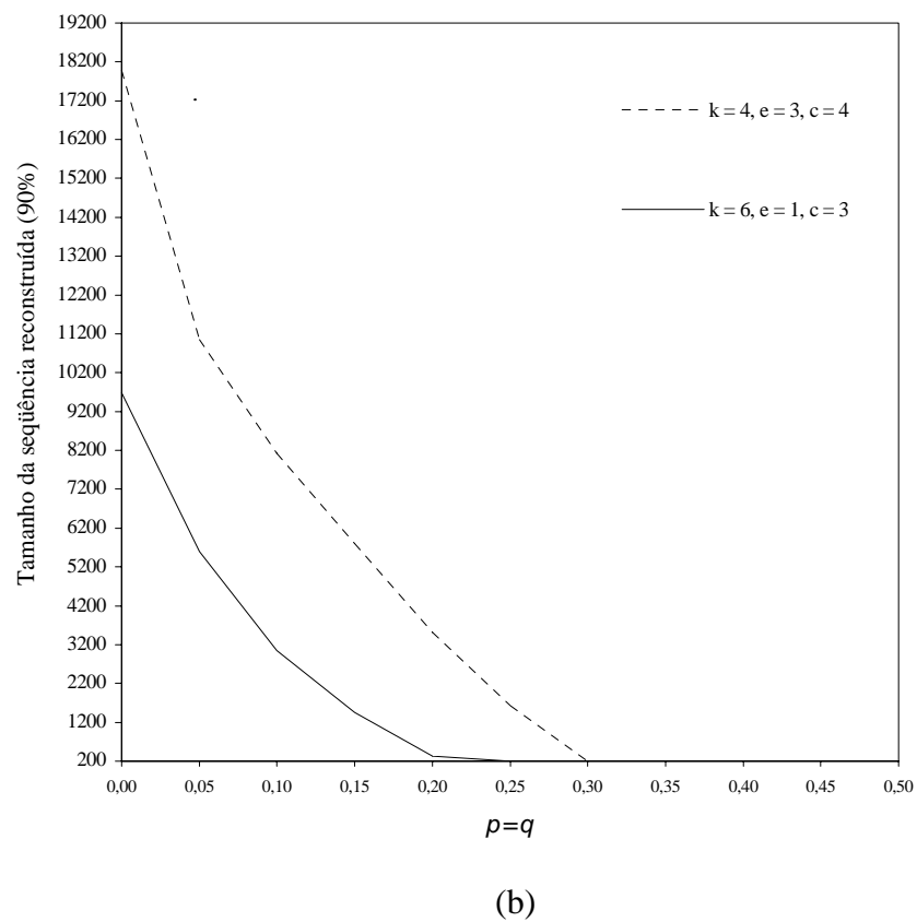
Figura 21A: Tamanho da seqüência corretamente reconstruída em aproximadamente 90% dos casos versus as taxas p e q ( p = q ) de erros, quando k + e = 7 , ck + e = 19 , (a) n = 4^8 e (b) n = 4^9 .
