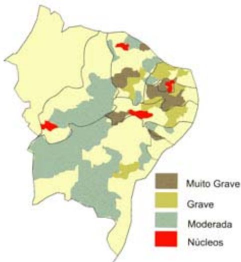
Figura 08: Mapa de distribuição de áreas susceptíveis ao fenômeno da desertificação no Nordeste brasileiro.
