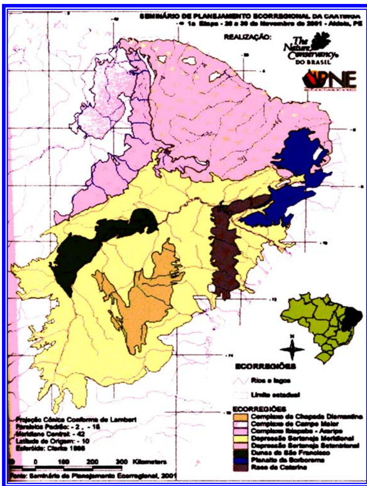
Figura 15: Delimitação das ecorregiões da caatinga. Fonte: VELLOSO et al., 2002.
