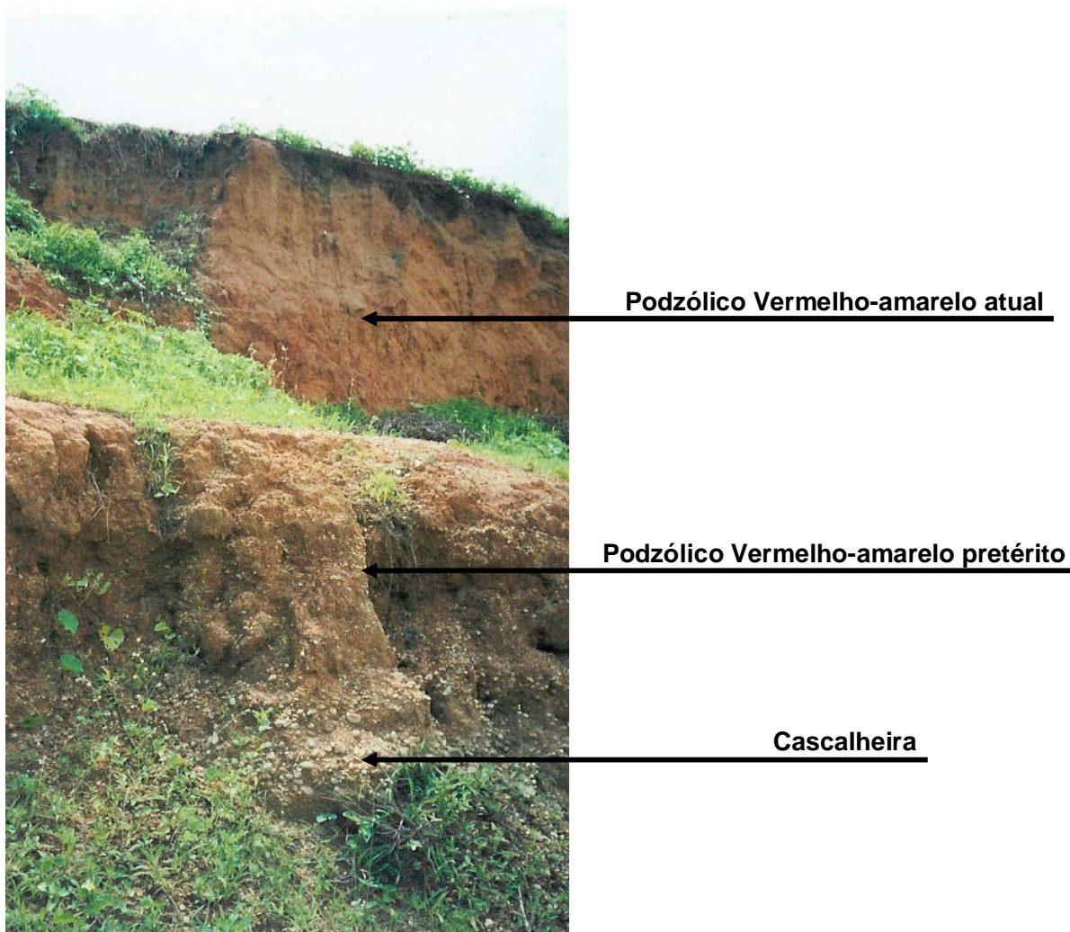
Figura 28: Aspecto do perfil de um solo tipo Podzólico vermelho-amarelo, no município de Tabuleiro do Norte – CE, com ocorrência de paleossolo Fonte: OLIVEIRA FILHO, Fevereiro/2003
