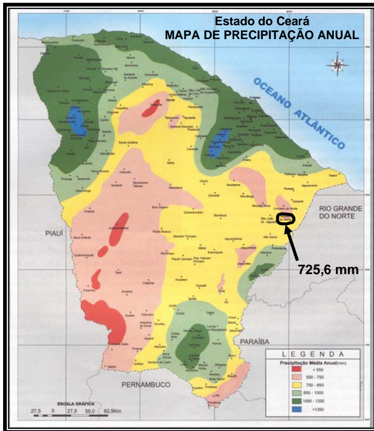
Figura 23: Mapa de Precipitação Média Anual do Estado do Ceará, com ênfase ao município Tabuleiro do Norte.
