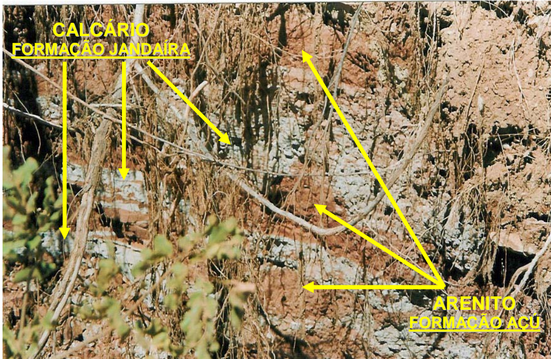
Figura 20: Fragmentos das unidades estruturais da chapada do Apodi: o Arenito (Formação Açu) e o Calcário (Formação Jandaíra).
