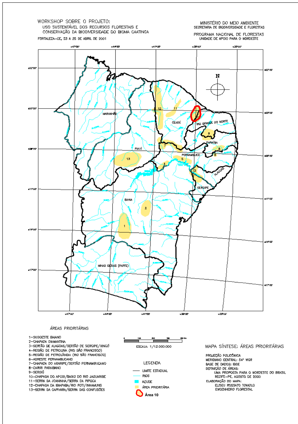
Figura 50: Mapa síntese das 13 áreas contempladas pelo projeto “Conservação da Biodiversidade e Uso Sustentável dos Recursos Florestais da Eco-região da Caatinga”, com ênfase a área 10.
