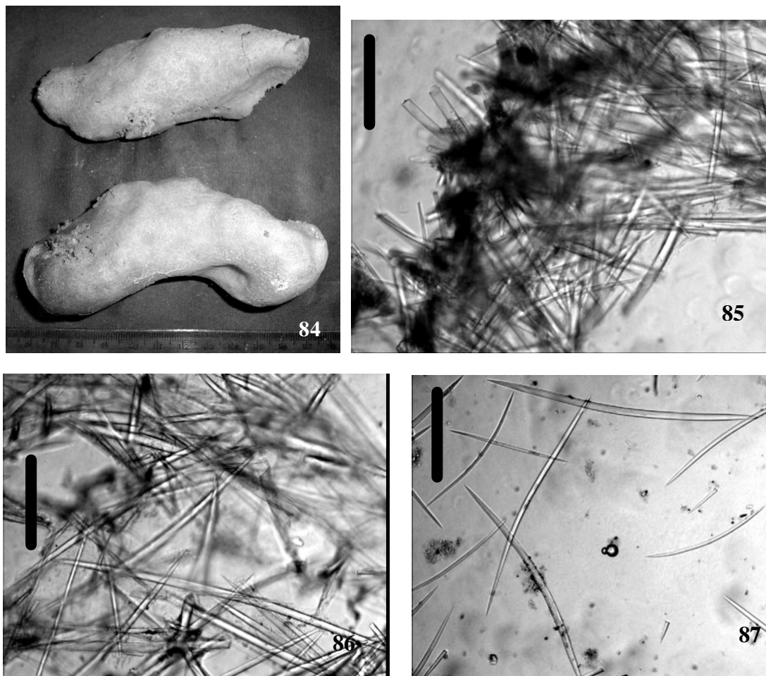
Figuras 84-87. Halichondria sp. 6. 84. Espécime fixado. 85. Corte perpendicular: ectossoma (Barra: 200 \mu m). 86. Corte perpendicular: coanossoma (Barra: 200 \mu m). 87. Escleras (Barra: 200 \mu m)
