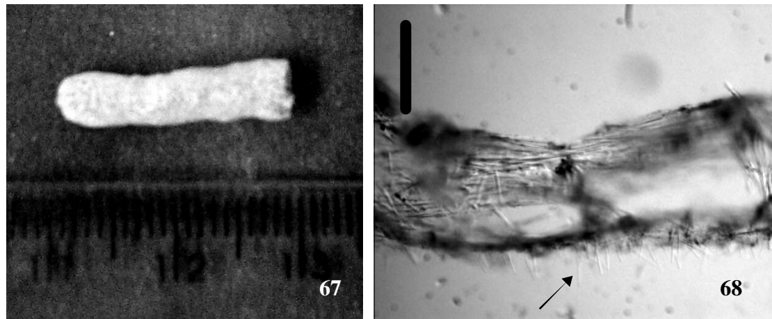
Figuras 67 e 68. Família Myxillidae sp. 67. Espécime fixado. 68. Corte perpendicular: Esqueleto coanossomal confuso, seta: acantóstilos protraem no ectossoma (Barra: 200µm).
