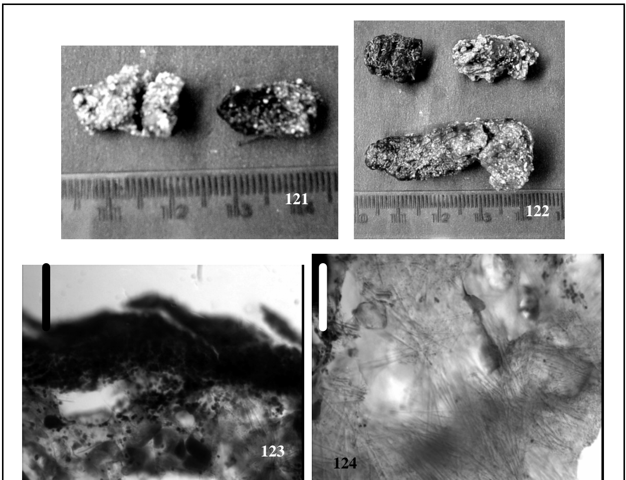
Figuras 121-124. Oceanapia sp. 2. 121 e 122. Espécimes fixados. 123. Corte perpendicularar: ectossoma (Barra: 100µm). 124. Corte perpendicularar: coanossoma (Barra: 200µm).
