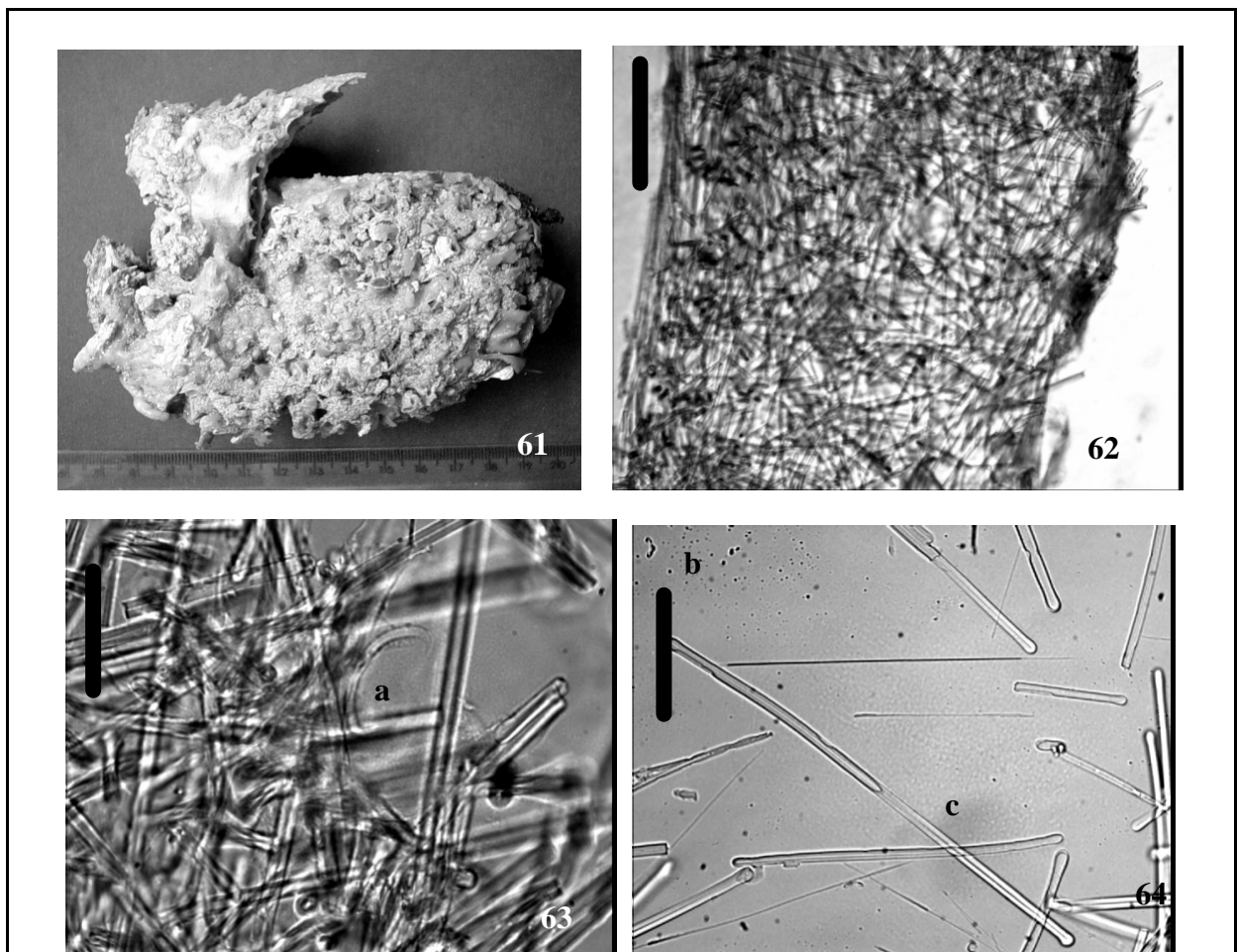
Figuras 61-64. Coelosphaera sp. 61. Espécime fixado. 62. Corte perpendicular (Barra: 100µm). 63. Corte perpendicular: a-sigma "C" (Barra: 400µm). 64. Escleras: b-estrôngilo, c-isoquela (Barra: 400µm).
