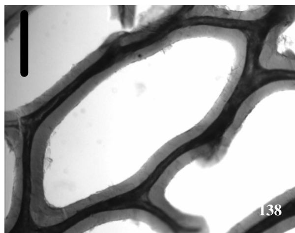
Figuras 137 e 138. Aplysina fistularis fulva (Pallas, 1766). 137. Espécime fixado. 138. Fibras medulares (Barra: 400 \mu m)
