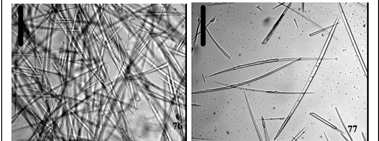
Figuras 74-77. Halichondria sp. 2. 74. Espécimes fixados. 75. Corte perpendicular com ectossoma (Barra: 200µm). 76. Corte perpendicular com coanossoma (Barra: 200µm). 77. Escleras: óxeas (Barra: 200µm).
