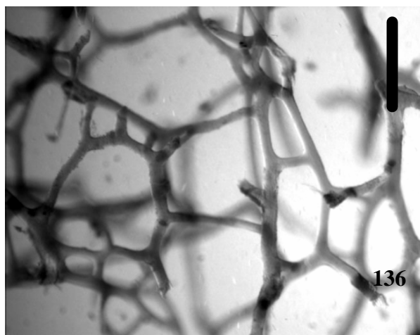
Figuras 135 e 136. Hyatella cavernosa (Pallas, 1766). 135. Espécime fixado. 136. Fibras (Barra:200 \mu m)
