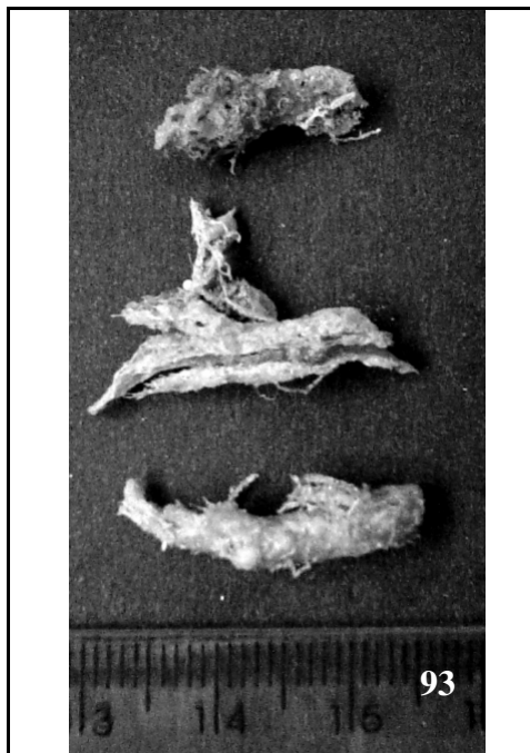
Figuras 93 e 94. Haplosclerida sp. 3.93. Espécime fixado. 94. Escleras (Barra: 200 \mu m).
