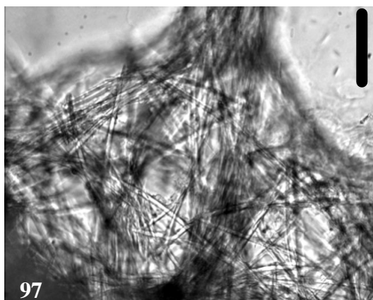
Figuras 95-98. Haplosclerida sp. 4. 95. Espécime fixado. 96. Corte perpendicular: coanossoma (Barra: 100 \mu m). 97. Corte perpendicular: detalhe do coanossoma (Barra: 200 \mu m). 98. Escleras (Barra: 200 \mu m)
