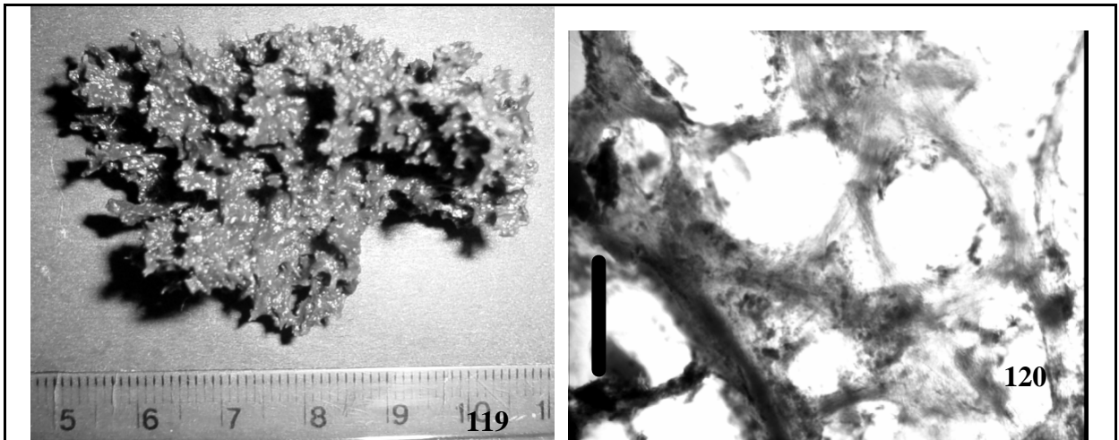
Figuras 119 e 120. Oceanapia sp. 1. 119. Espécimes fixados. 120. Corte perpendicularar: coanossoma (Barra: 200µm)
