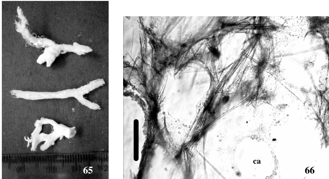
Figuras 65 e 66. Monanchora sp. 65. Espécimes fixados. 66. Corte perpendicular: coanossoma, ca- canal aquífero (Barra: 200µm).
