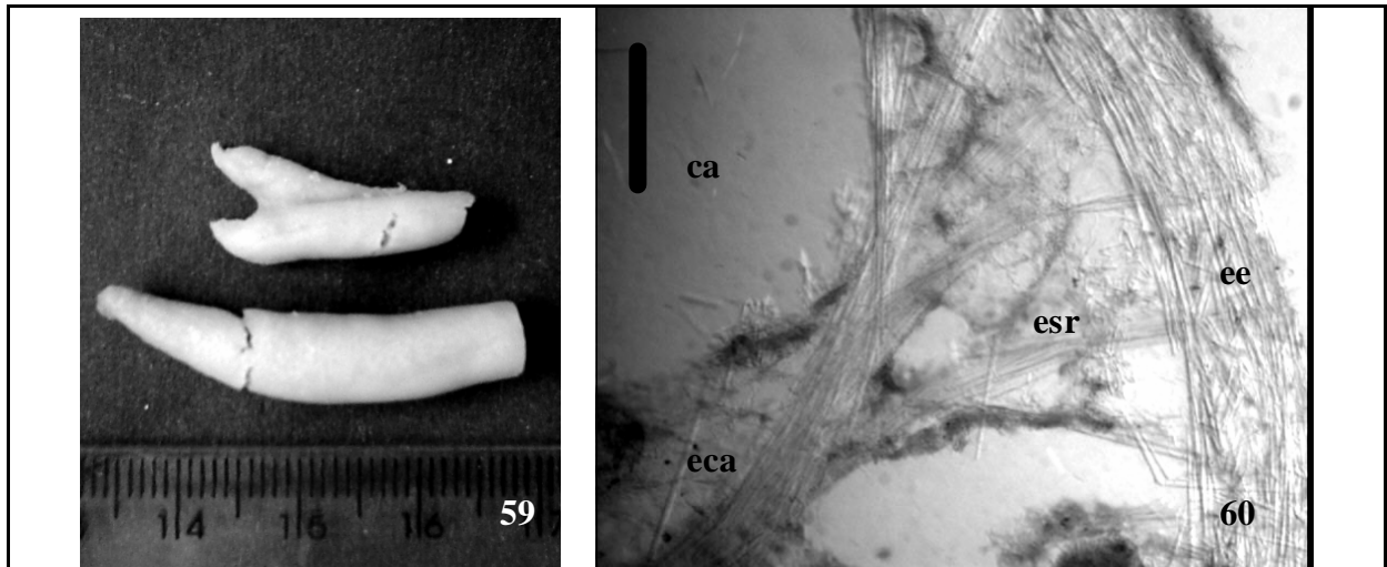
Figura 59 e 60. Mycale (Mycale) quadripartita (Boury-Esnault, 1973). 59. Espécime fixado. 60. Corte perpendicular: ca-canal aquífero, eca-esqueleto central axial, esr-esqueleto secundário radial, ee-esqueleto ectossomal .
