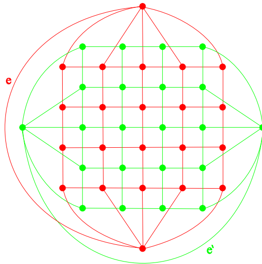
Figura 4.1. Grafo associado ao jogo Bridge-it( n = 4 ) mais a aresta e , e seu dual.
