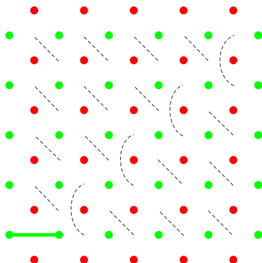
Figura 1.3. A estratégia de Oliver Gross. Observe que, como está posicionado o tabuleiro, o primeiro jogador joga objetivando ligar um ponto da esquerda a um da direita.
