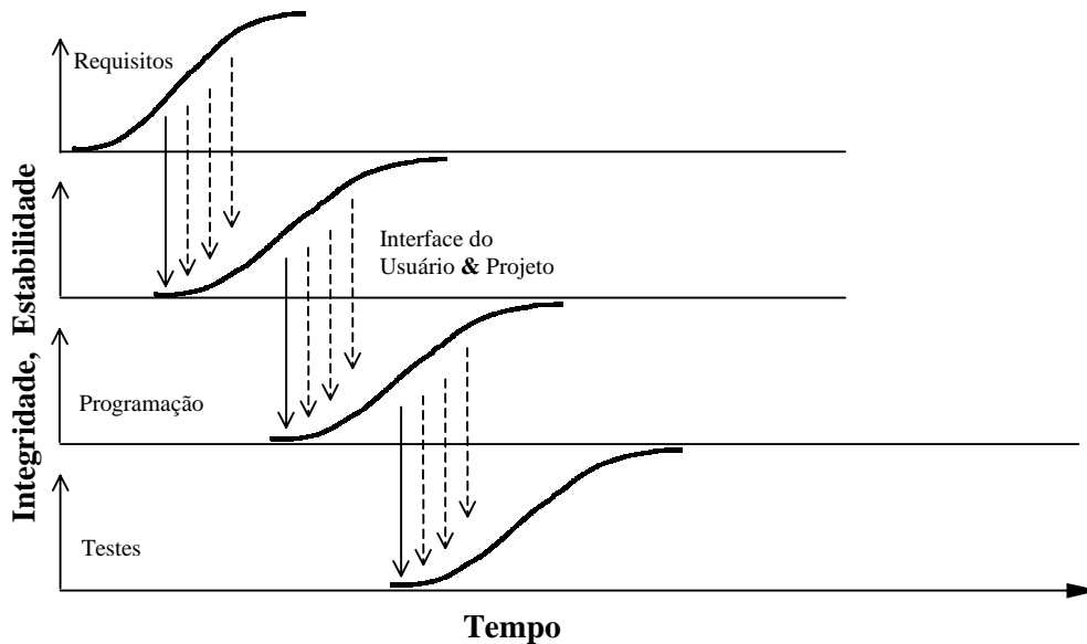
Figura 2.11 – Um Desenvolvimento Concorrente.
