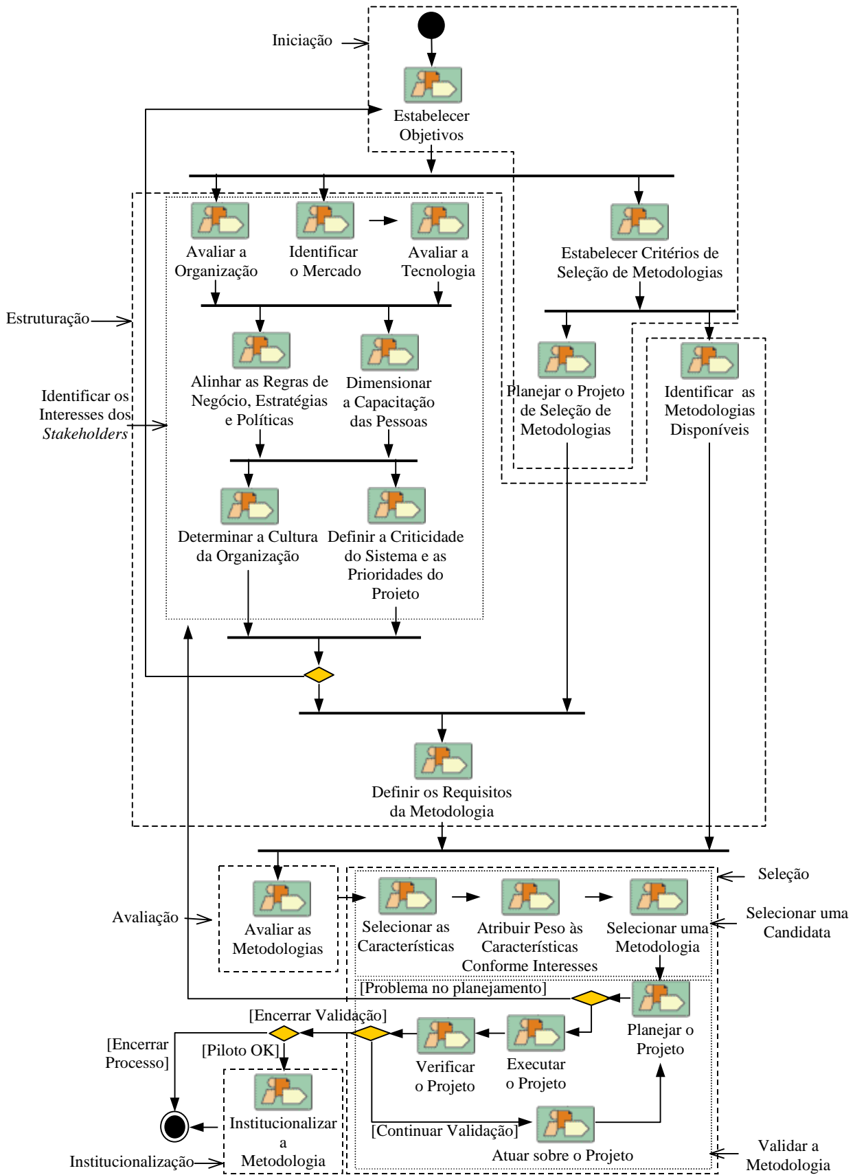
Figura 4.9 – As Atividades do Processo Proposto.
