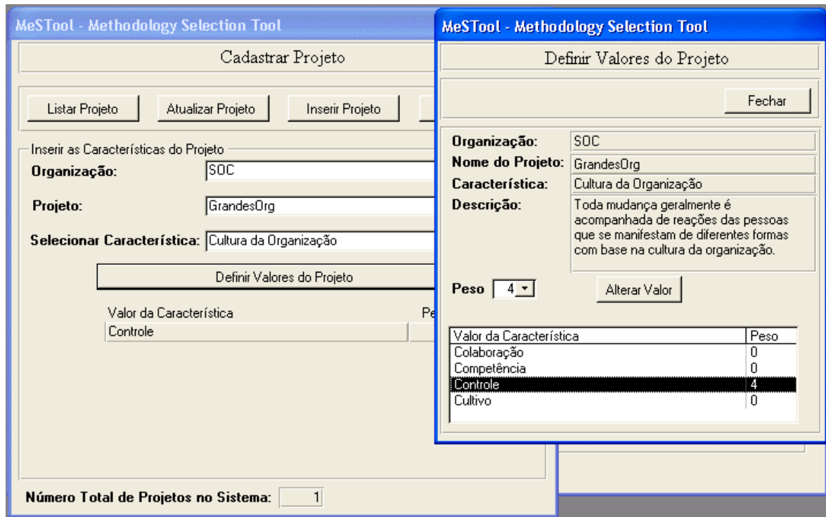
Figura 5. 18 – Definir Valores de uma Característica no Projeto.
