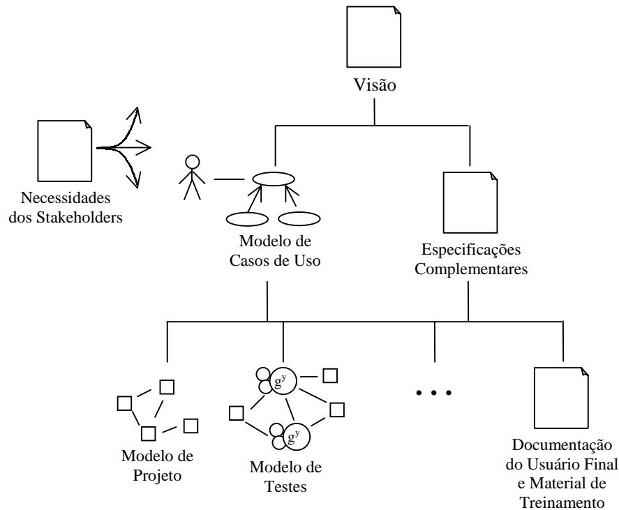
Figura 2. 2 – Principais Artefatos do RUP.
