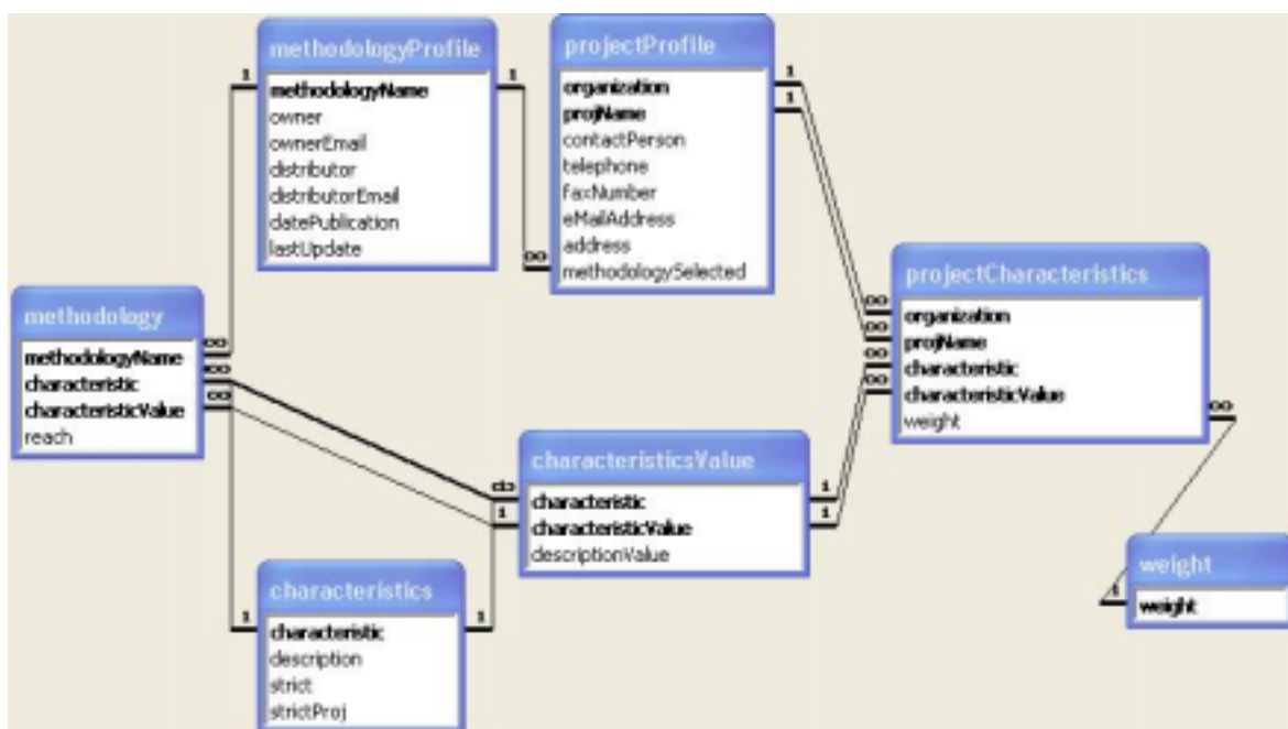
Figura A. 2 – O Modelo de Dados Conceitual do MeSTool.
