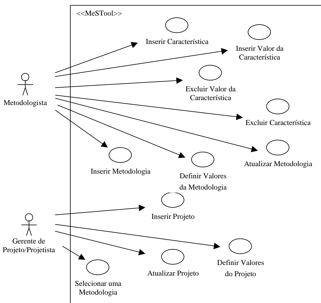
Figura A. 1– Os Casos de Uso.
