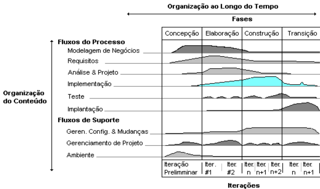
Figura 2. 1 – A Arquitetura do RUP com Duas Dimensões.
