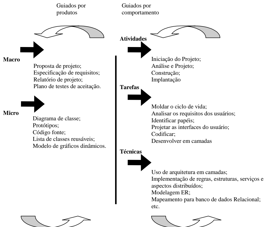
Figura 2. 15 – O Planejamento de um Projeto em OPEN.
