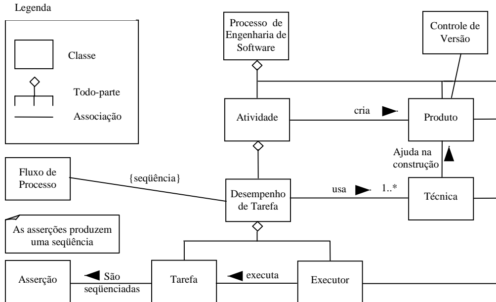
Figura 2. 4 – Atividades, Tarefas e Técnicas.
