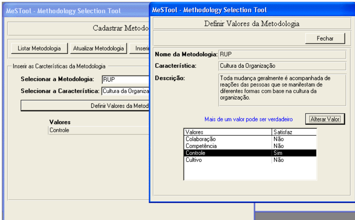
Figura 5.12 – Definir Valores da Metodologia.
