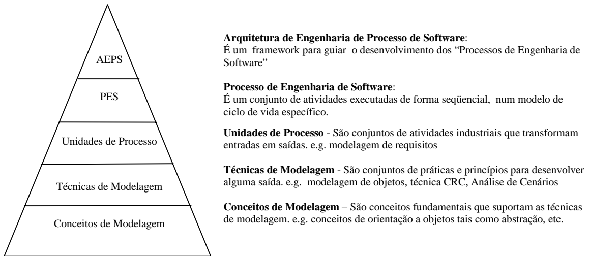
Figura 2. 3 – O Conceito Fundamental que Suporta o Process e-MeNtOR e o Próprio OPEN.
