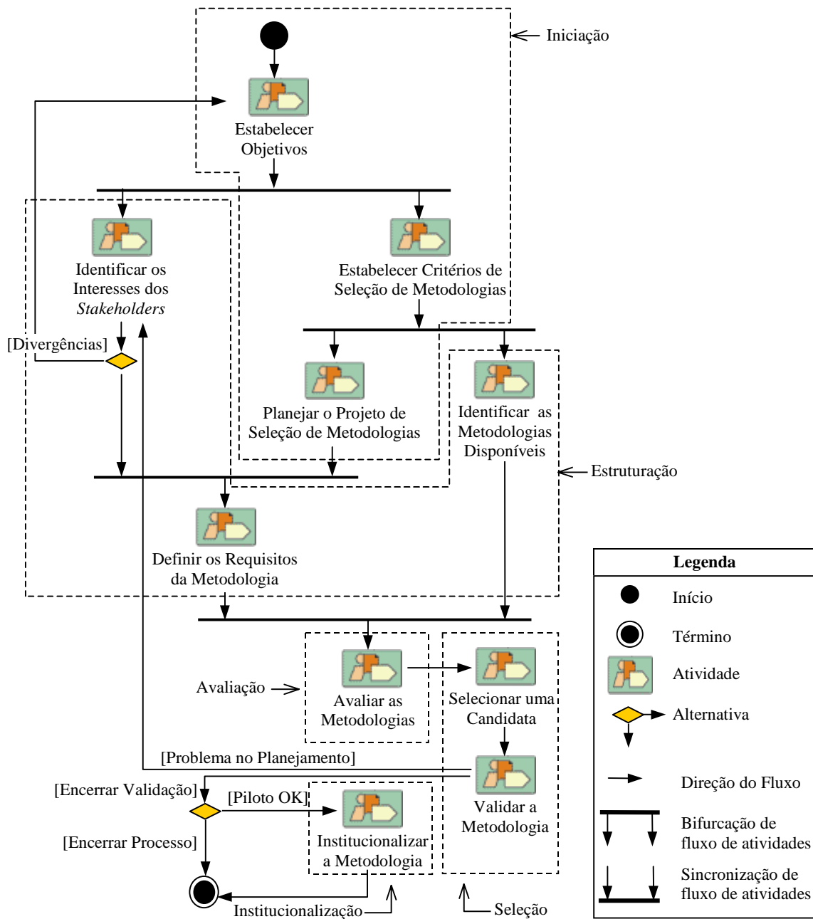
Figura 4. 1– A Proposta de uma Solução para a Seleção de Metodologias.
