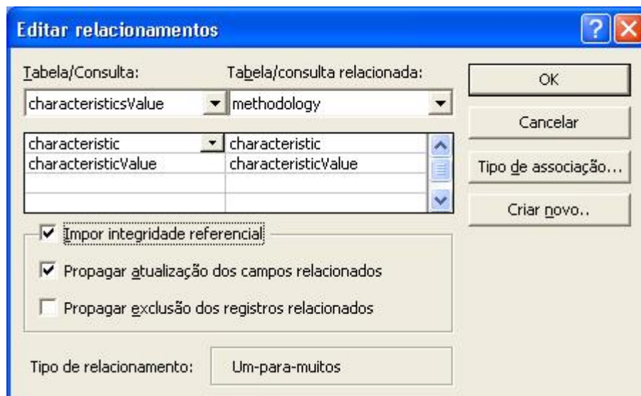
Figura A. 3 – A Janela Editar Relacionamentos.
