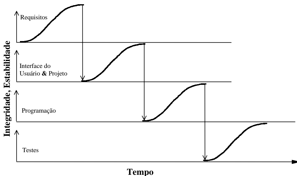
Figura 2.10 – Um Desenvolvimento Serial.
